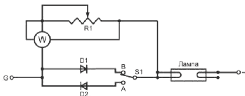
Рисунок Н.2 — Схема испытаний асимметричной мощностью
