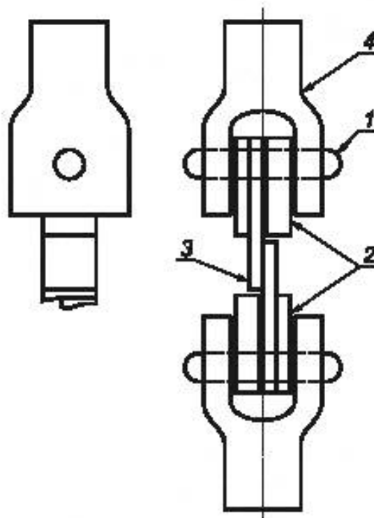
1 — осевая шпонка; 2 — разделительная прокладка; 3 — соединенный образец; 4 — вилка
