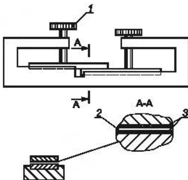
1 — винт с накатанной головкой; 2 — клей; 3 — покрытие
