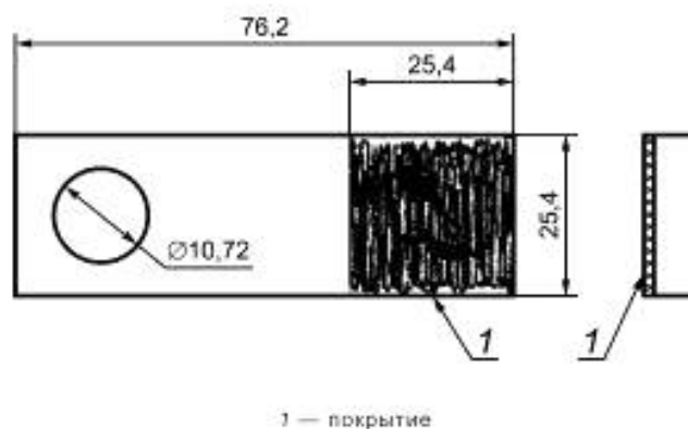
Рисунок 7 — Образец покрытия для испытания на сдвиг (только для металлических покрытий)
