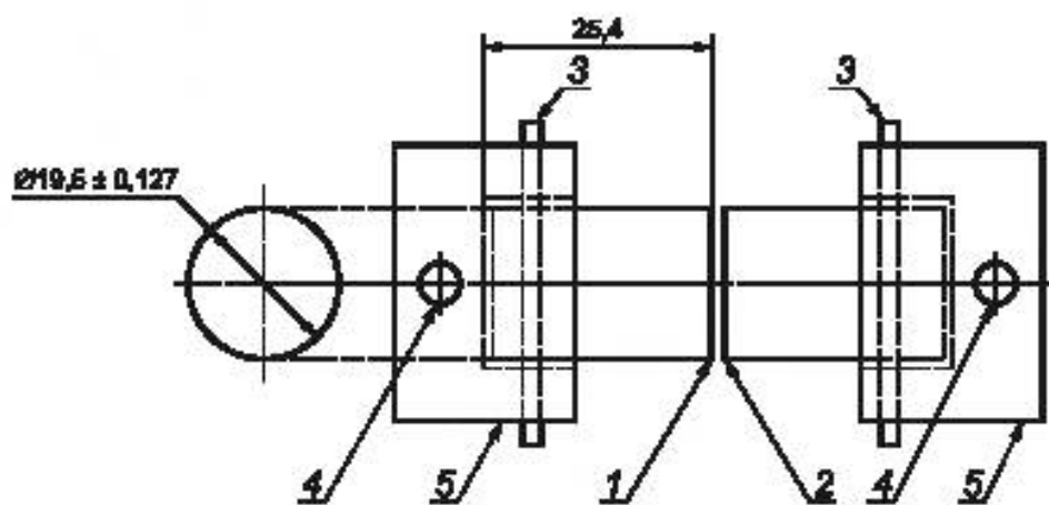
1 — покрытие (гидроксилалпатит); 2 — клей; 3 — осевая шпонка; 4 — отверстия для крепления сборки в испытательной машине; 5 — металлические стаканы для крепления образцов
