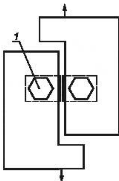
1 — шестигранный болт
