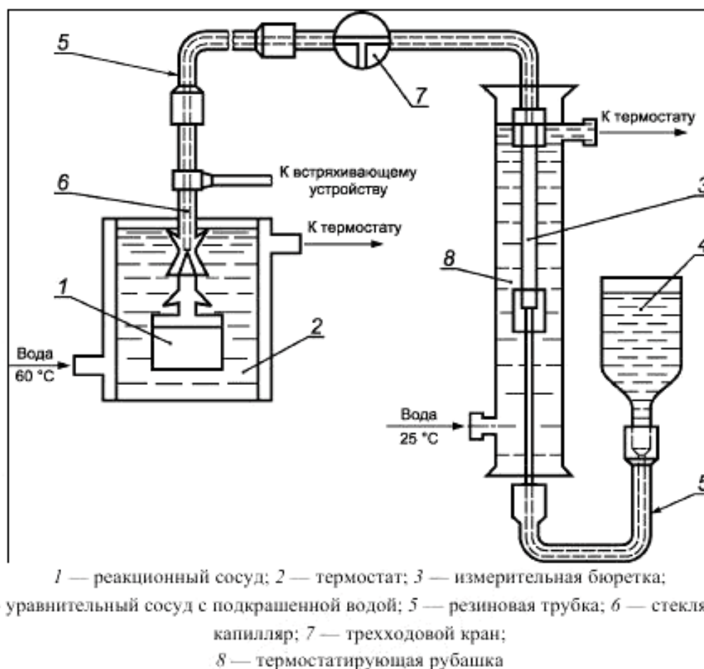
Рисунок 1 — Газометрическая установка
