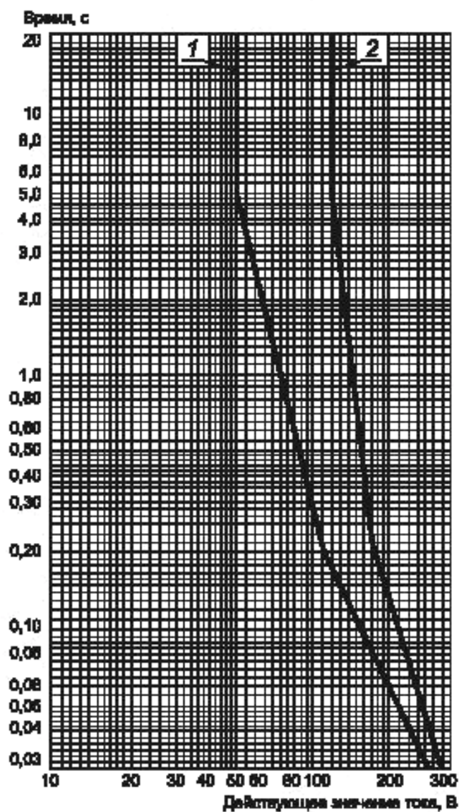
Рисунок С.1 — Кривая продолжительности предполагаемого напряжения прикосновения в соответствии с таблицей С.1
