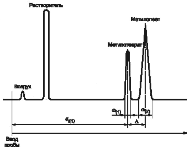
Рисунок А.1 — Хроматограмма для определения количества теоретических тарелок колонки (эффективности) разрешающей способности
