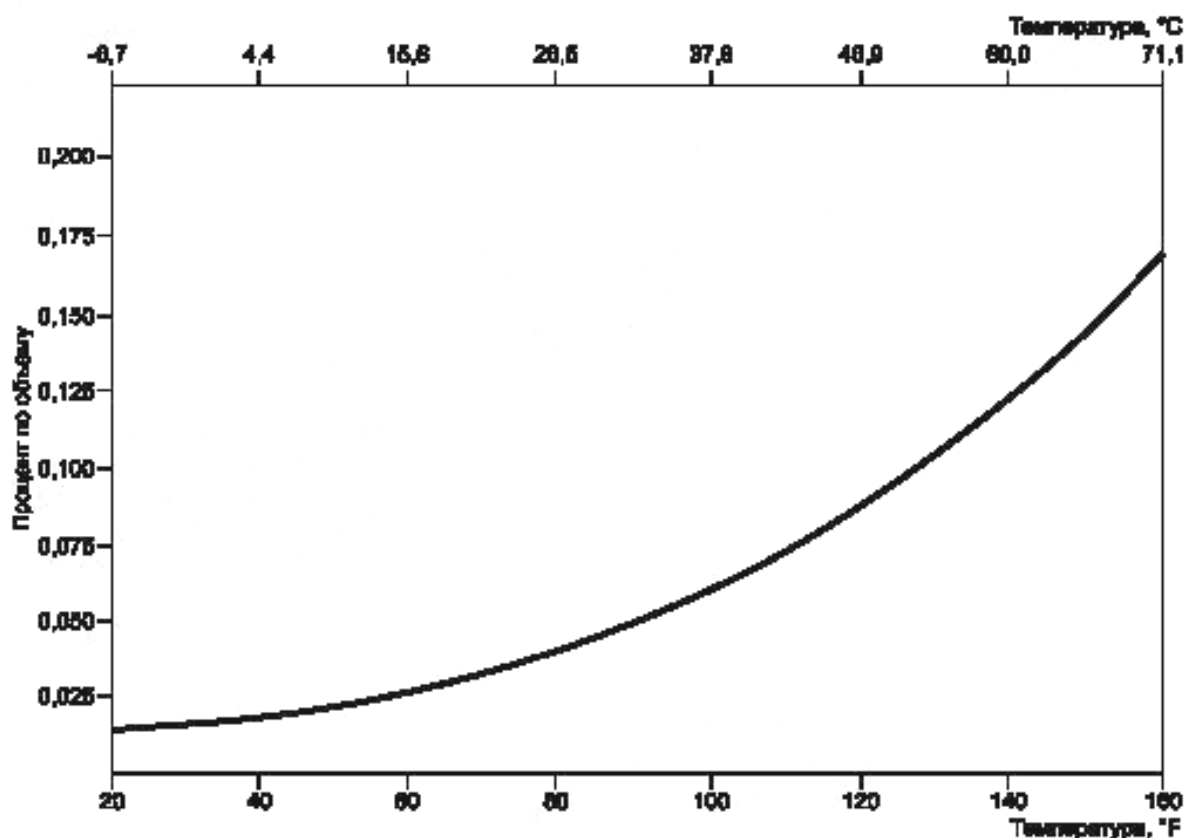
Рисунок А.1.1 — Растворимость воды в толуоле
