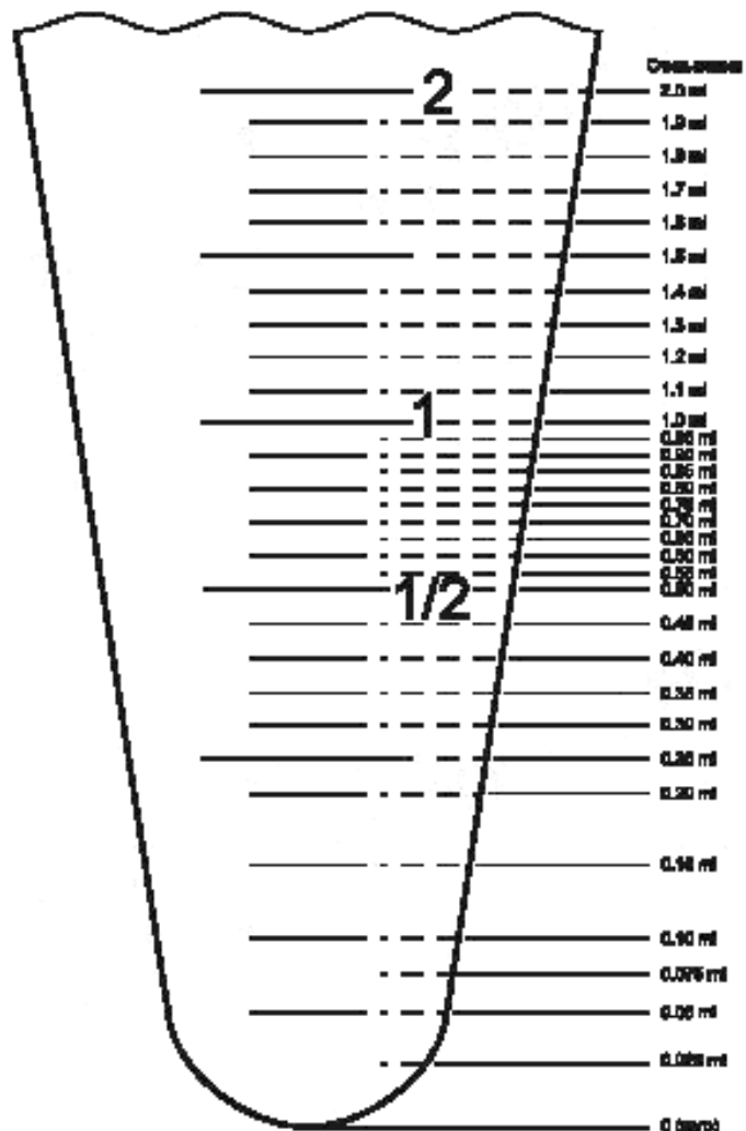
Рисунок 2 — Снятие показаний содержания воды и осадка при использовании конической пробирки для центрифугирования ASTM вместимостью 100 мл
