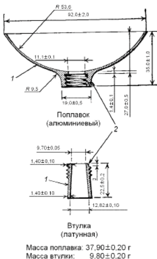
Рисунок 1 – Устройство поплавкового типа (поплавок)
