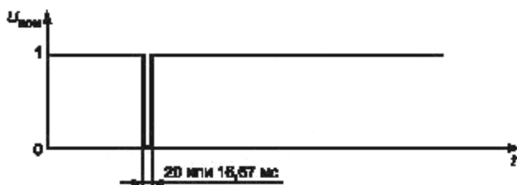
Рисунок В.2 — Прерывания напряжения \Delta U = 100\% , в течение одного цикла при номинальной частоте
