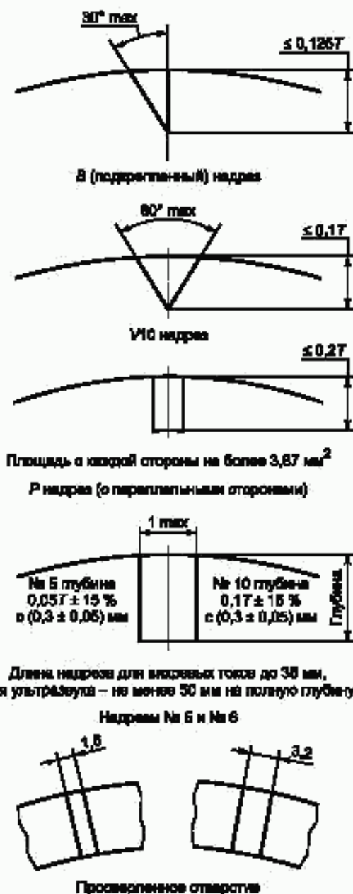
Рисунок 10 — Эталонные образцы (8.10.11.3.2)
