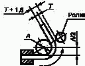
Конструкция с обкаткой роликом
