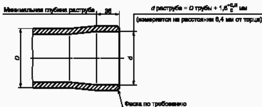
Рисунок 2 — Раструбный конец для соединения труб между собой
