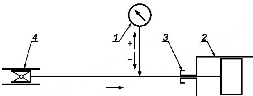
1 — циферблатный индикатор; 2 — поршень; 3 — устройство для прижимного уплотнения; 4 — кресткопф.
