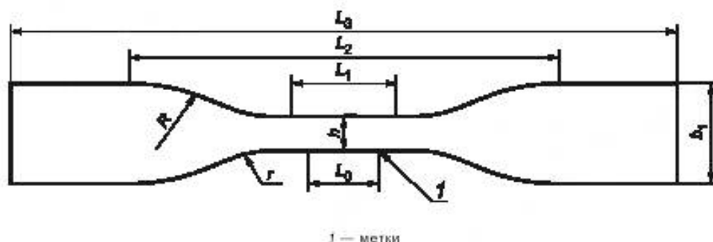
Рисунок 2 — Образец-лопатка (метод В)
