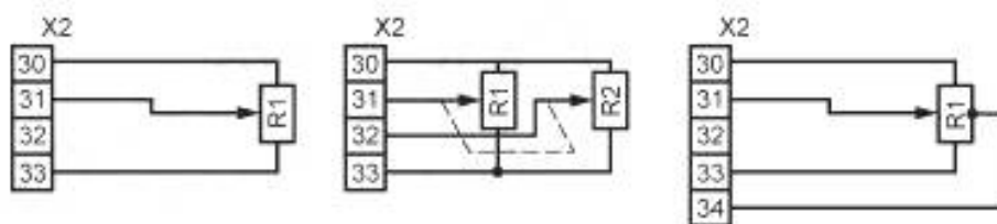
Схема подключения резистивных датчиков
