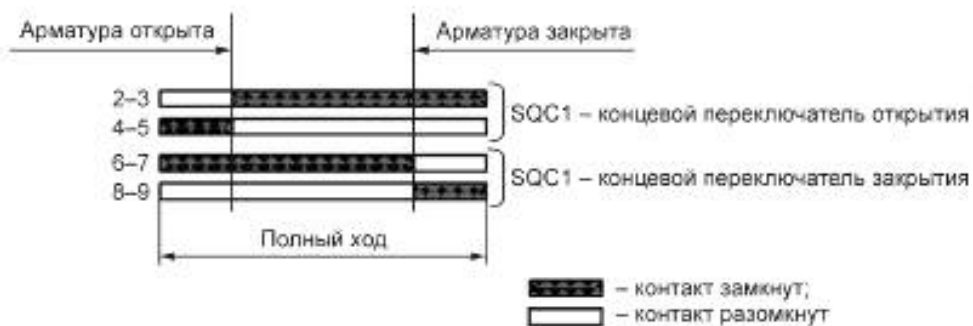
Рисунок У.1 — Электрическая схема соединения конечных переключателей арматуры с ручным управлением
