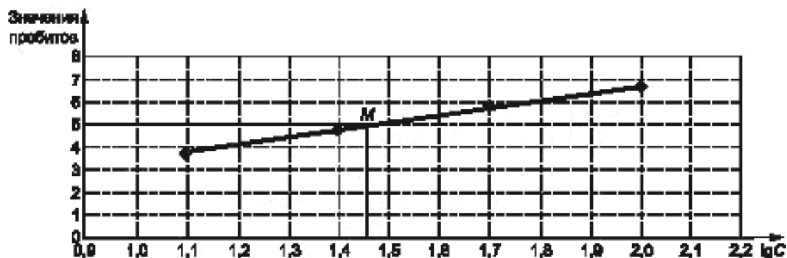
Рисунок Д.Б.1 – График линейной зависимости значений пробитов от lg С анализируемой пробы сточной воды
