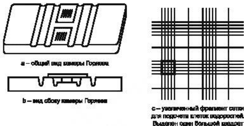
Рисунок Д.В.1 – Счетная камера Горяева
