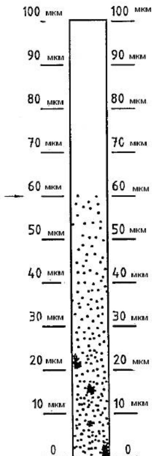
Рисунок 3 – Вид прибора с испытанным образцом
