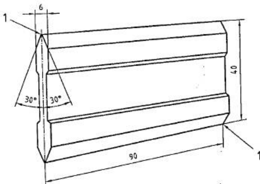
1 – лезвие скребка R 0,25 Рисунок 2 – Скребок
