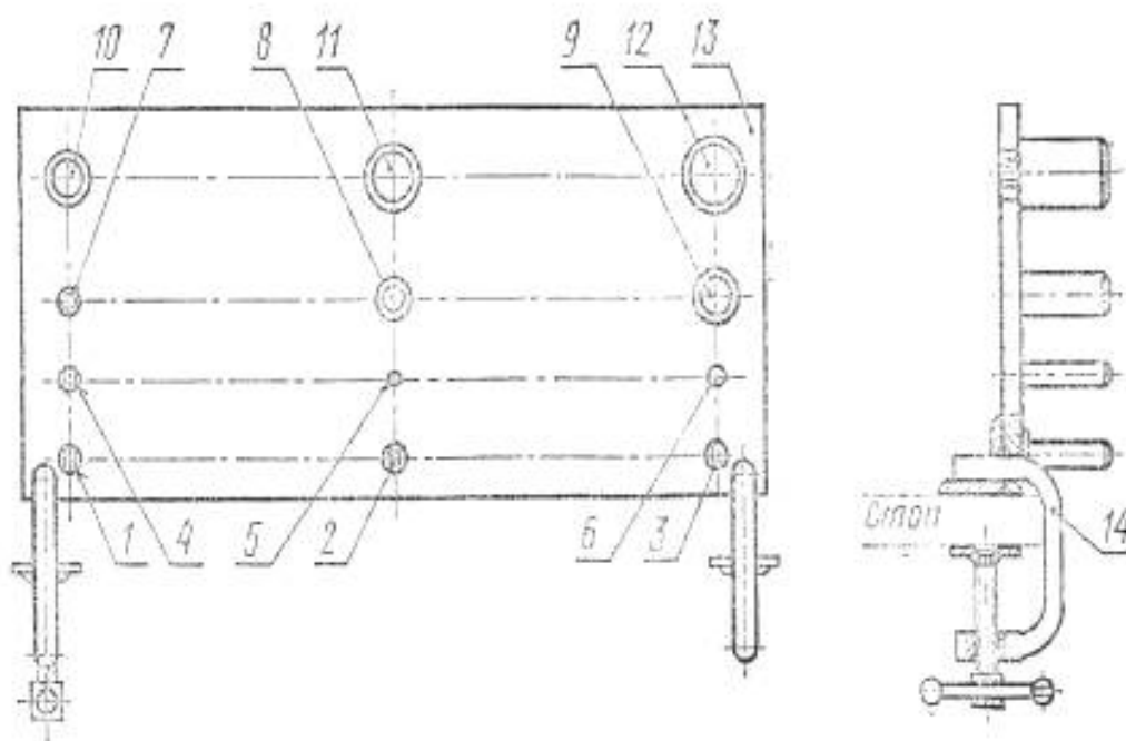
1– 12 – стержни; 13 – панель; 14 – струбцина; 15 – стол
