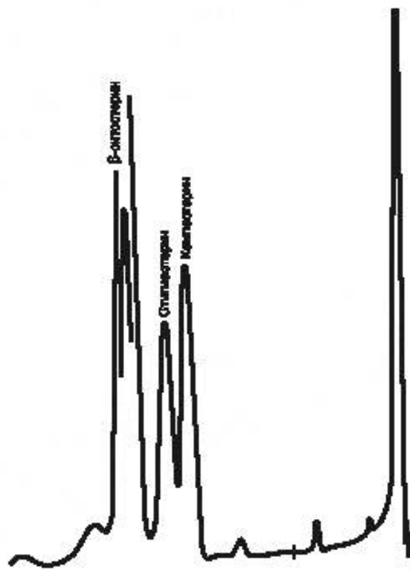
Рисунок А.3 — Хроматограмма стерина соевого масла
