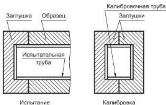
а) Средства испытаний с калиброванными заглушками
