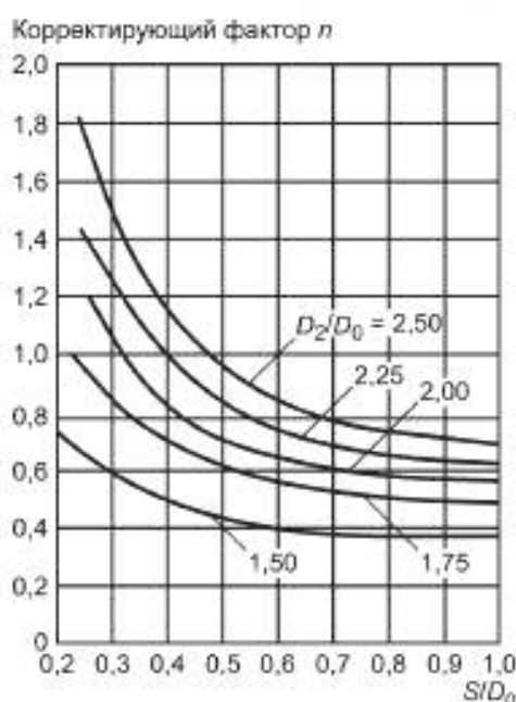
Рисунок 3 — Корректировка по методу Нукиямы
