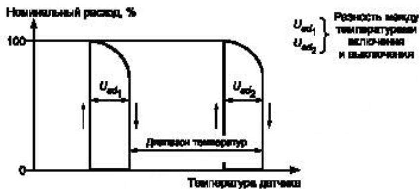
б) Двухпозиционный терморегулятор
