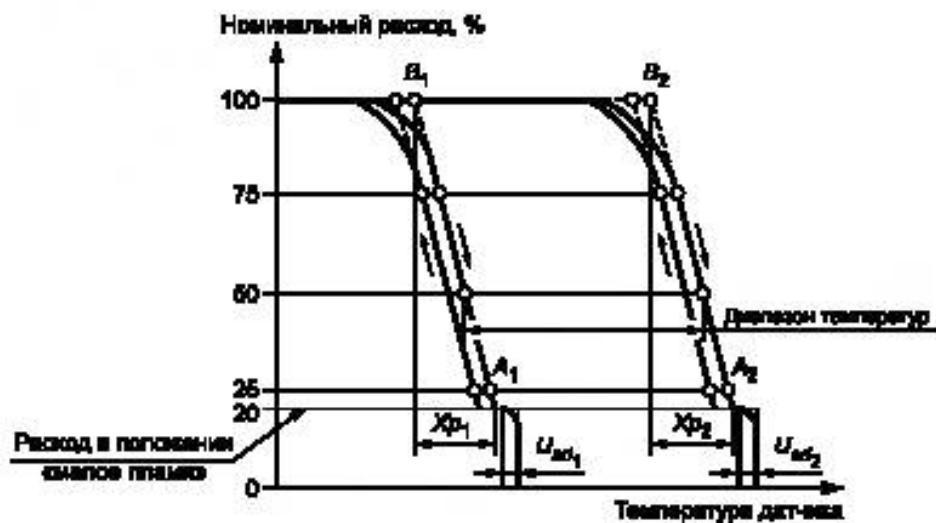
с) Терморегулятор непрерывного действия с двухпозиционным режимом работы
