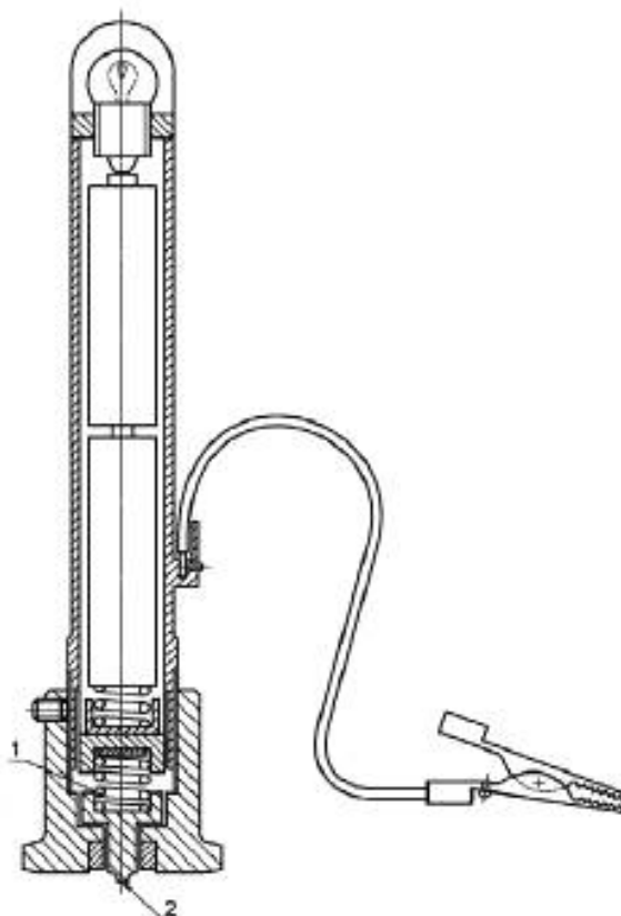
Рисунок 9 — Приспособление для проверки механической прочности лакокрасочного покрытия
