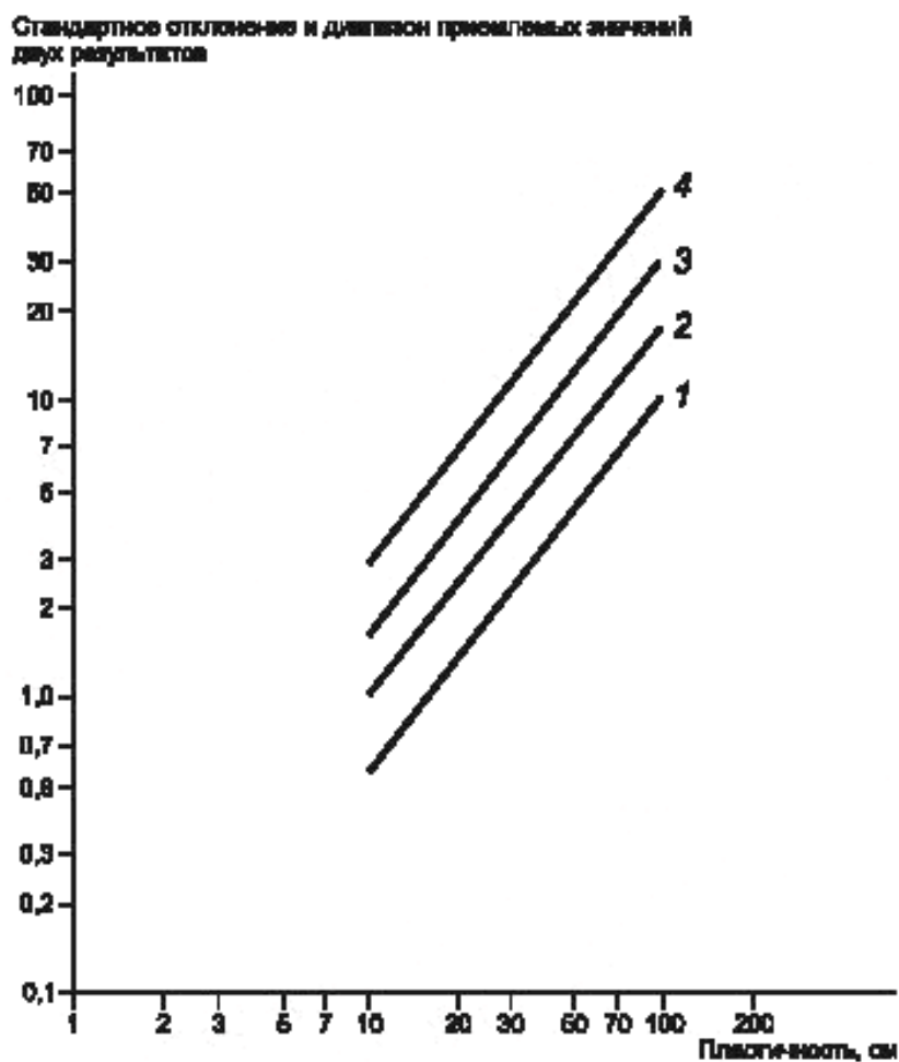
Рисунок 2 — Данные прецизионности
