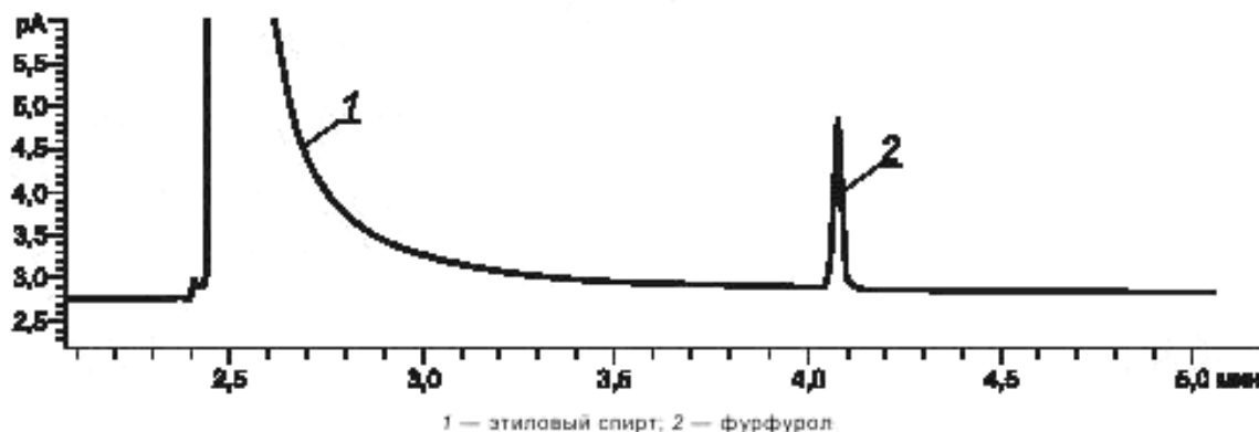
Рисунок 2 — Хроматограмма анализа градуировочной смеси на содержание фурфурола
