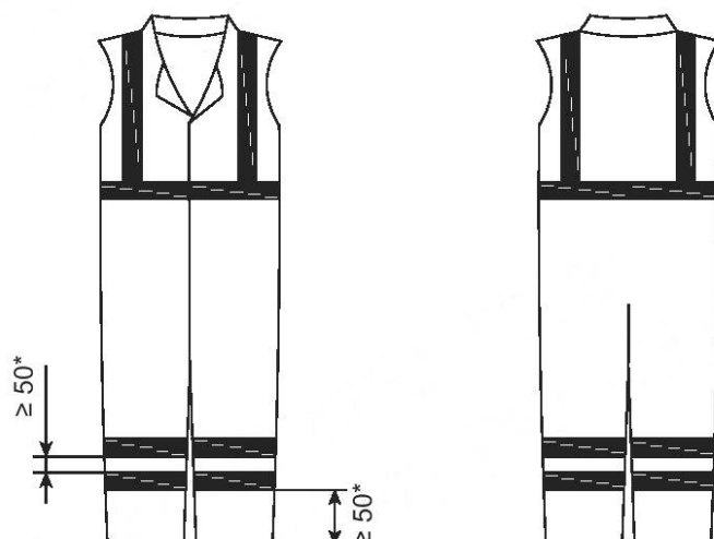
Рисунок А.3 — Расположение световозвращающих сигнальных элементов на предметах одежды, покрывающих ноги
