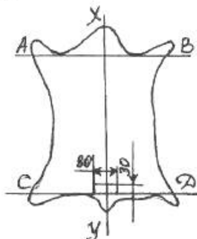
Рисунок 3 - Схема расположения образцов для определения светостойкости окраски
