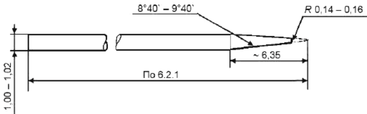
Рисунок 1 – Игла для определения пенетрации
