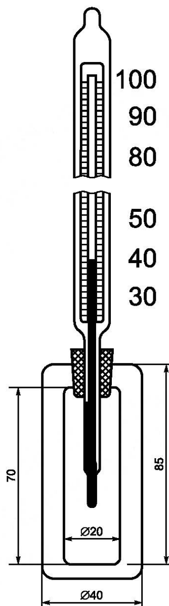
Рисунок 1 — «Прибор Жукова»
