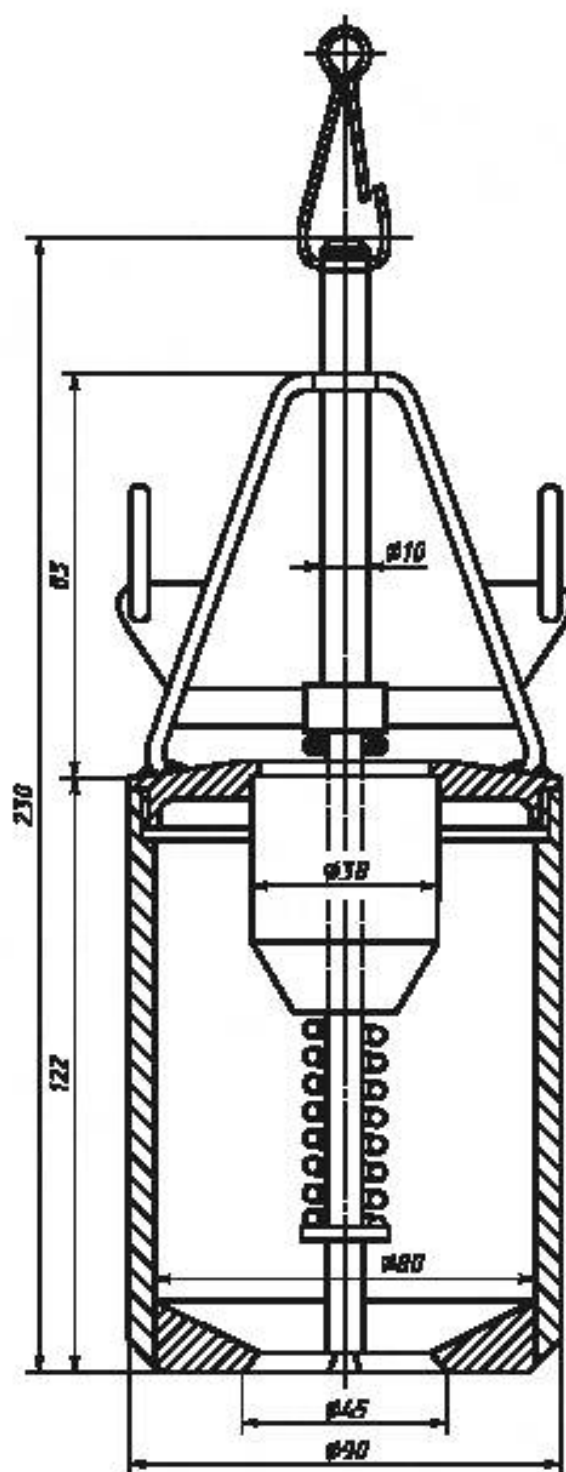
Рисунок А.2 — Зональный пробоотборник
