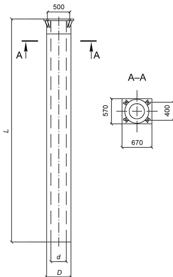
Рисунок 46 — Свая цилиндрическая фланцевая.
