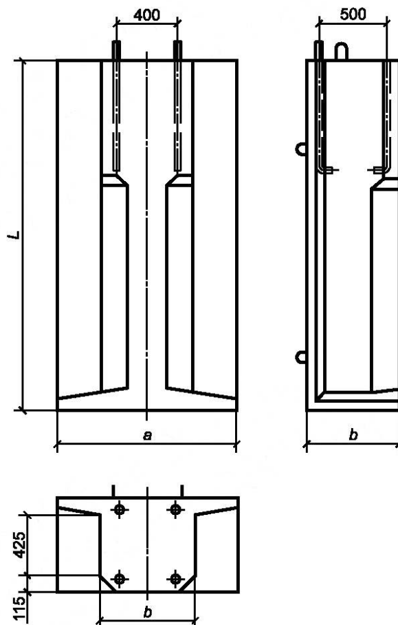
Рисунок 4 — Фундамент с уширенной полкой
