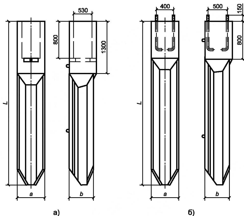
Рисунок 1 — Трехлучевые фундаменты: а) со стаканом креплением стоек; б) с анкерным креплением стоек
