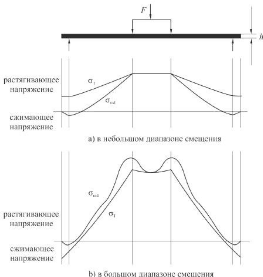
Рисунок 1 – Схема зависимости радиального и тангенциального напряжений от радиуса образца в процессе нагрузки устройством двойного кольца
