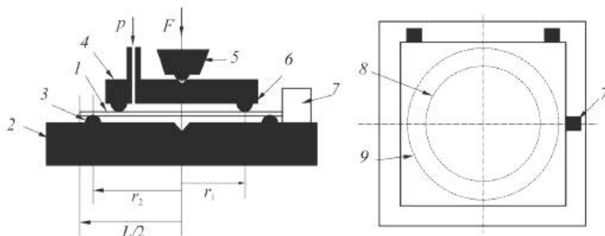
Рисунок 2 – Нагрузочное устройство
