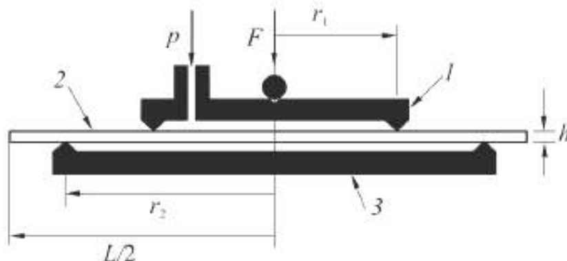
Рисунок 1 – Основная схема оборудования для испытаний 1 – нагрузочное кольцо; 2 – образец; 3 – опорное кольцо
