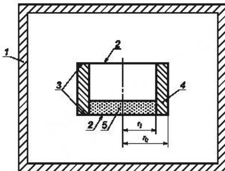
Рисунок 1 — Схема испытания по определению характеристик паропроницаемости
