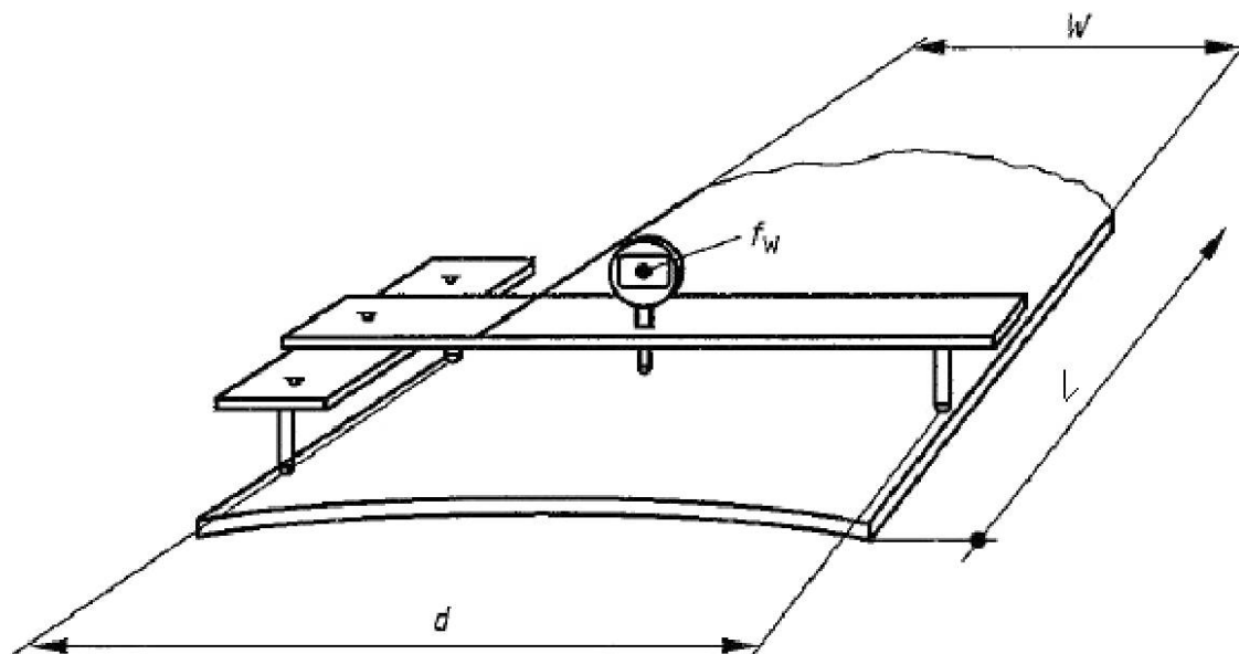
Рисунок А.6— Определение покоробленности по ширине f_w
