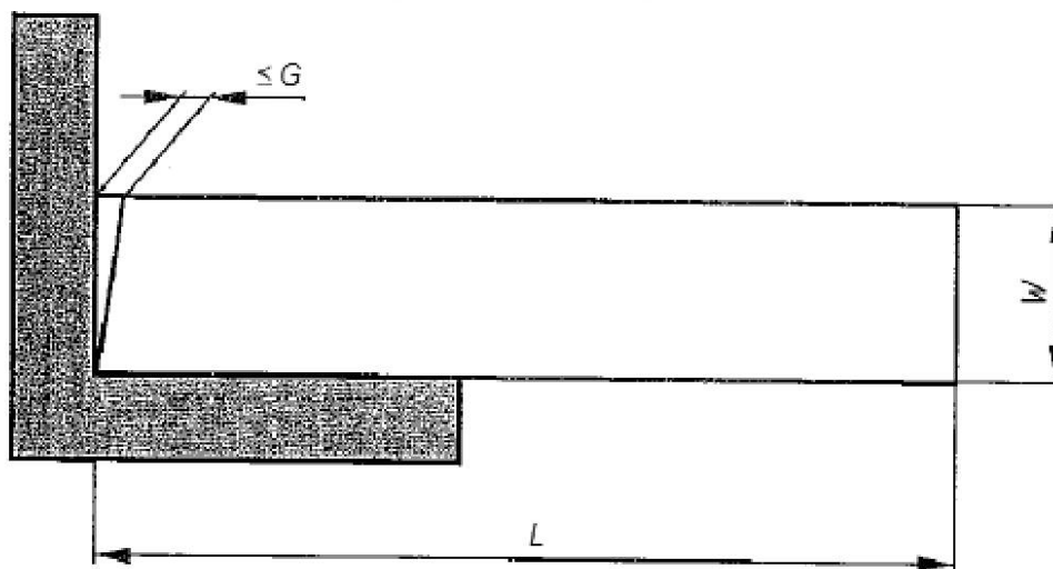
Рисунок А.4— Определение прямоугольности G
