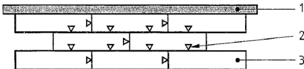
1 – проверочная линейка; 2 – точки приложения щупа индикаторного глубиномера в местах соединения элементов напольного покрытия; 3 – образец для испытания
