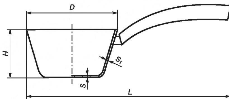
Рисунок 7 — Ковш
