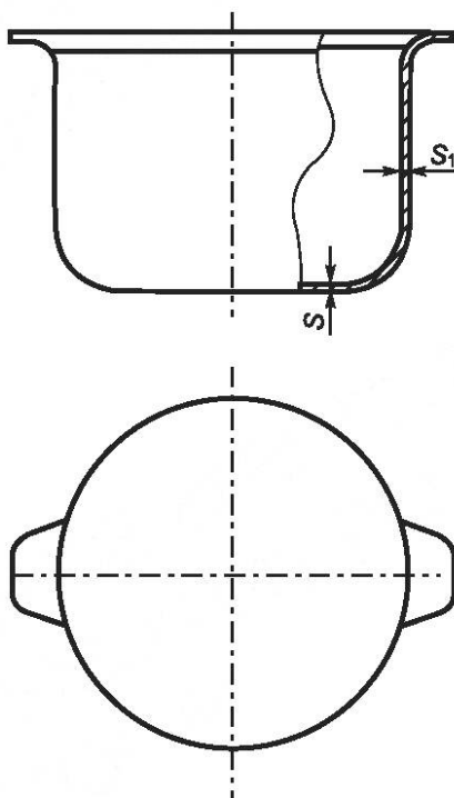
Рисунок 11 — Котел
