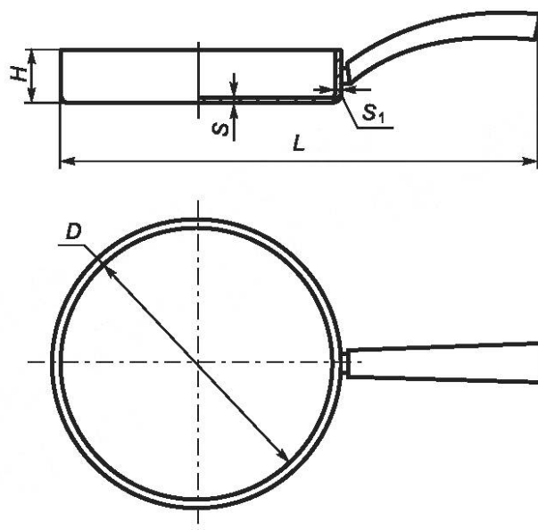
Рисунок 5 — Сотейник с одной ручкой
