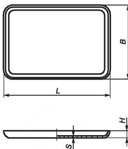
Рисунок 9 — Противень
