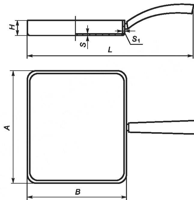
Рисунок 4 — Квадратная сковорода с одной ручкой
