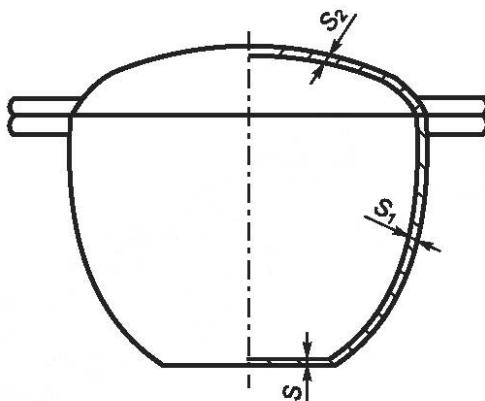
Рисунок 8 — Казан
