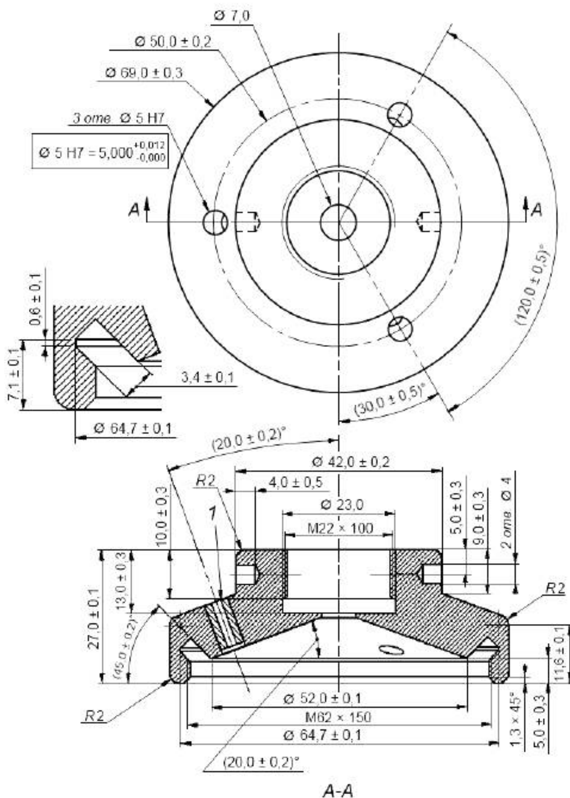
Рисунок 3 – Крышка
