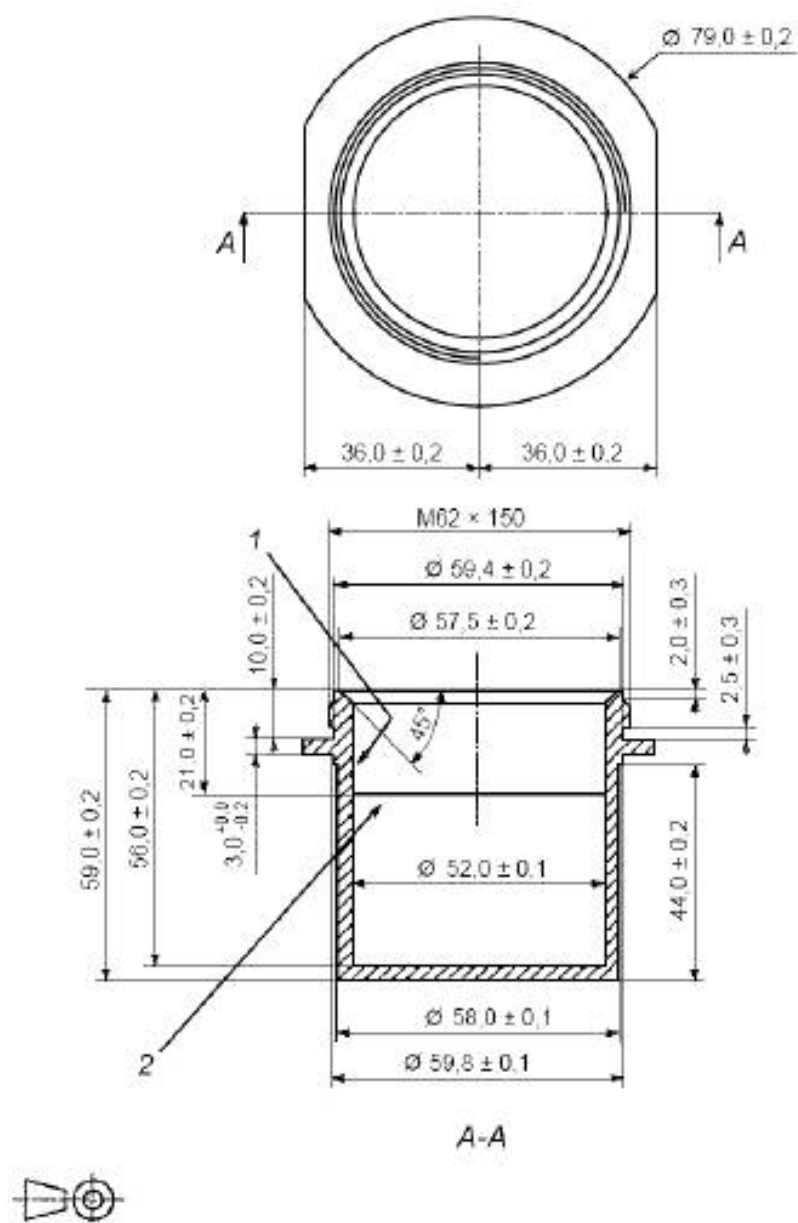
Рисунок 2 – Тигель из нержавеющей стали
