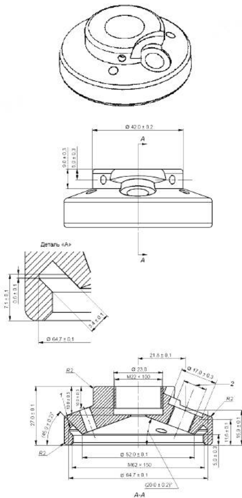
Рисунок 9, Лист 1 – Крышка тигля (деталь 2 на рисунке 7)
