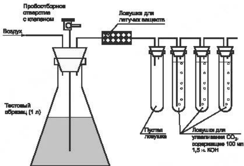
Рисунок А.1 — Пример проточной испытательной установки
