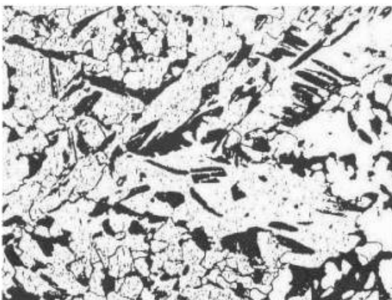
Кратность увеличения 500 ×
