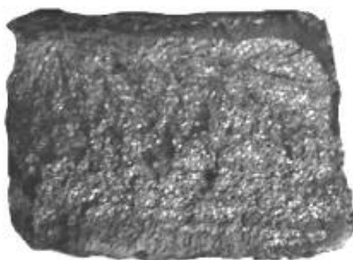
Рисунок Б.11 — Излом мелкозернистый, кристаллический
