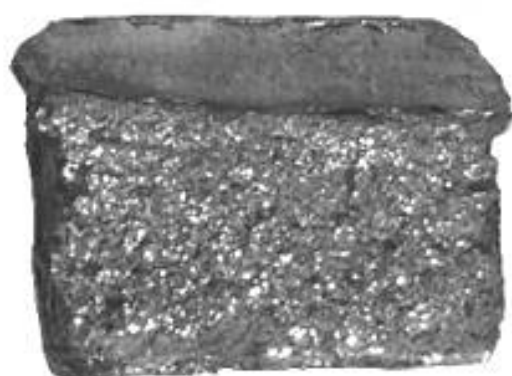
Рисунок Б.13 — Излом среднезернистый, кристаллический
