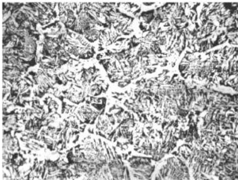
Кратность увеличения 100×
