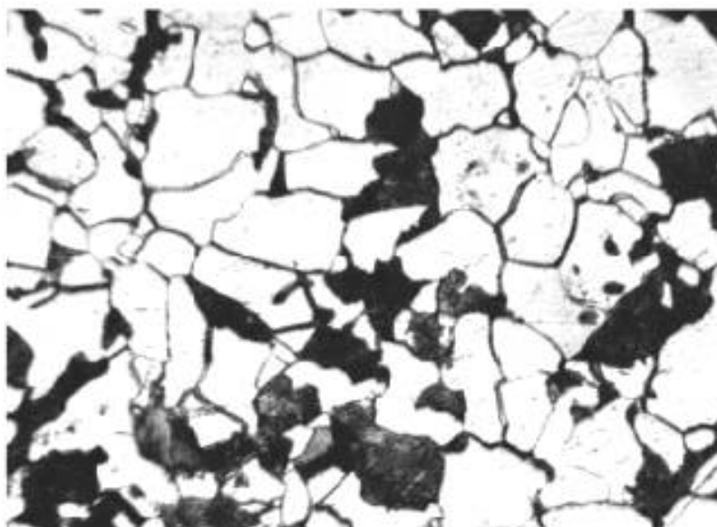
Кратность увеличения 500×
