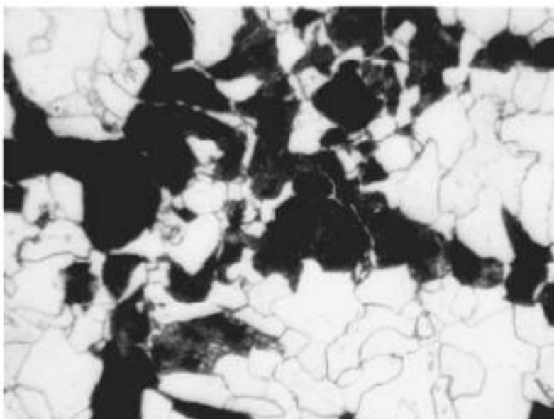
Кратность увеличения 500×
