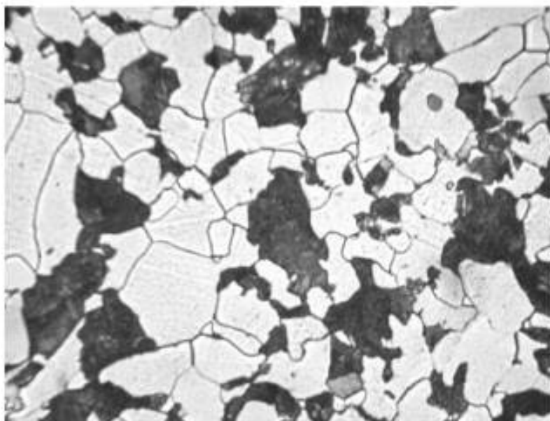
Кратность увеличения 500×
