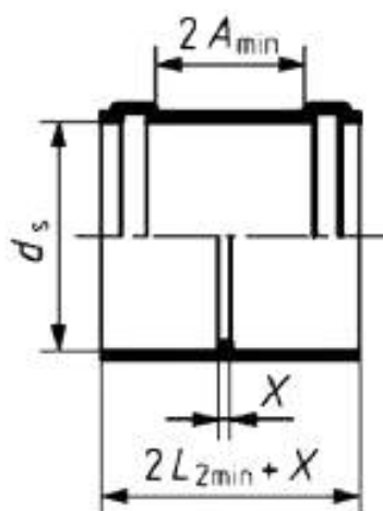
Рисунок 7 – Муфта
