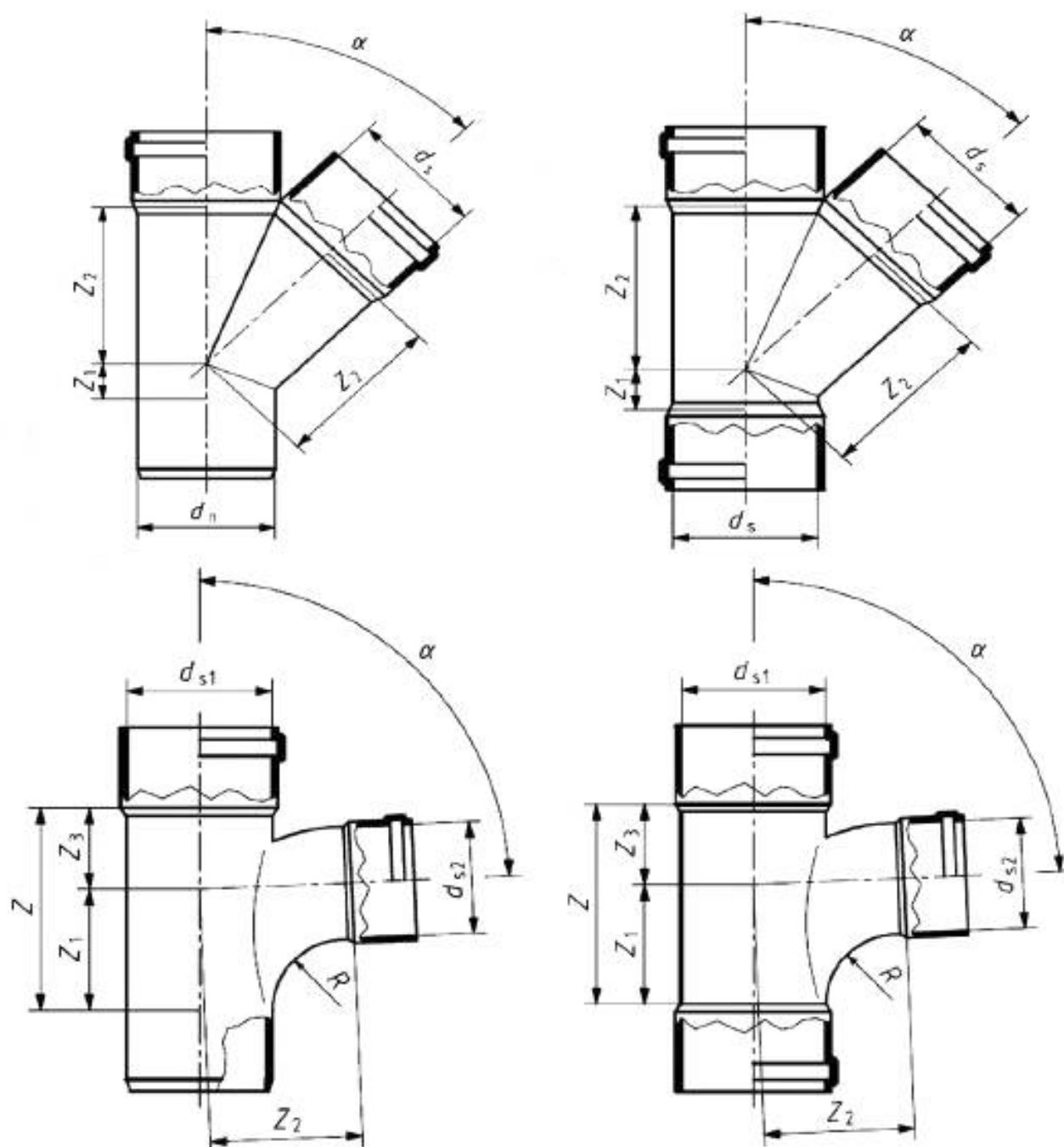
Рисунок 9 – Тройник
