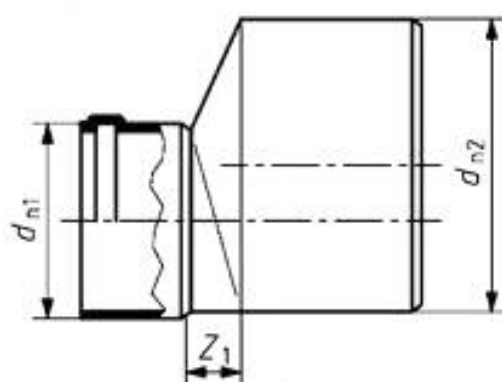
Рисунок 8 – Патрубок переходной
