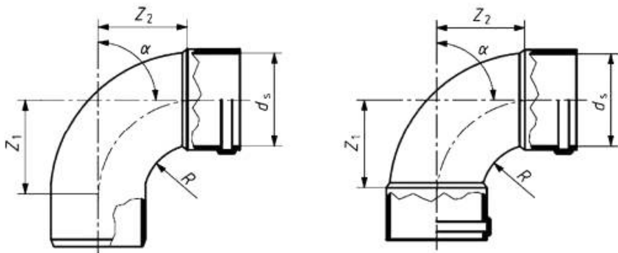
Рисунок 6 – Отвод
