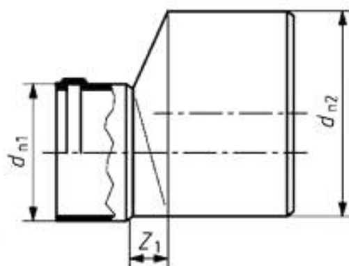
Рисунок 8 – Патрубок переходной
