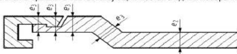
Рисунок 4 – Толщина стенки раструба с крышкой для установки уплотнительного кольца
