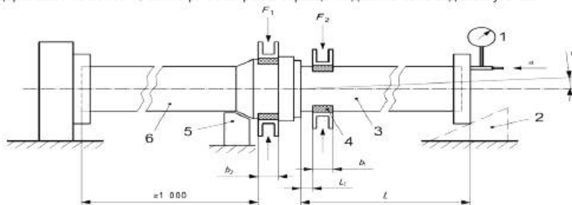
1 – манометр или вакуумметр; 2 – регулируемая опора для создания осевого смещения; 3 – труба или трубный конец фасонной части; 4 – зажимы; 5 – фиксатор раструба; 6 – труба или фасонная часть с раструбом; а – подключение к источнику давления
