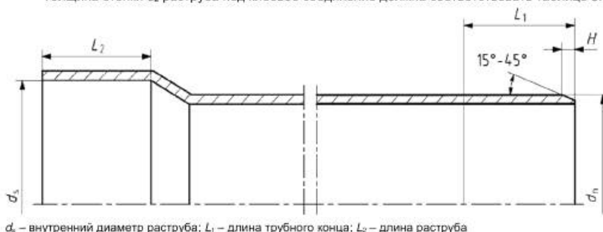
Рисунок 5 – Основные размеры раструба и трубного конца под клеевое соединение
