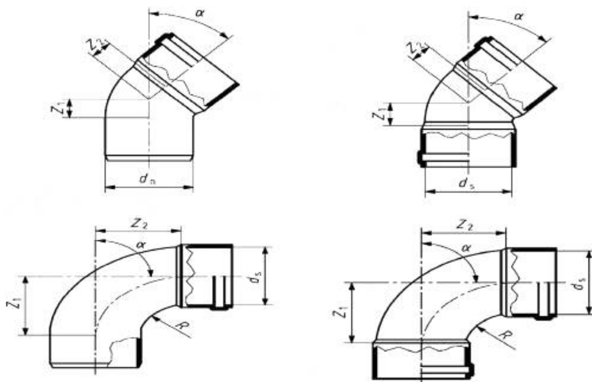
Рисунок 6 – Отвод
