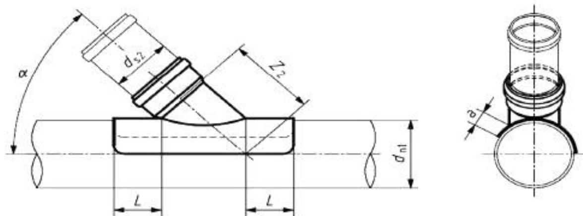
Рисунок 10 – Седловой отвод
