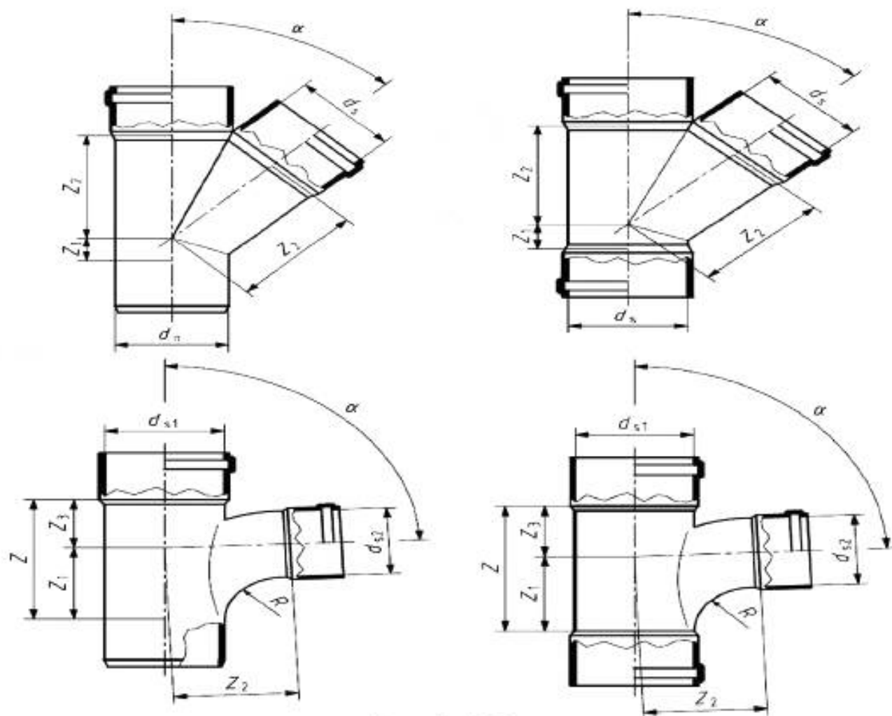
Рисунок 9 – Тройник
