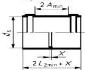
Рисунок 7 – Муфта
