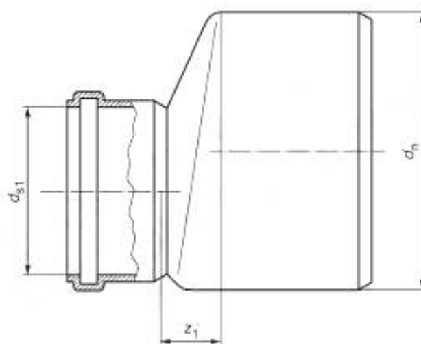
Рисунок 7 — Патрубок переходной
