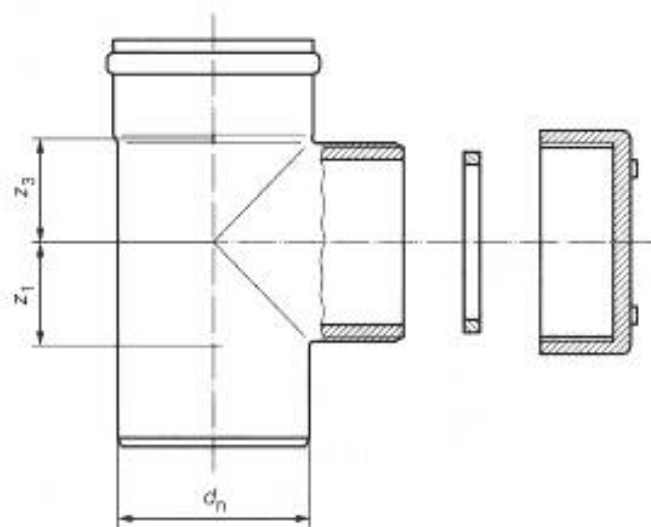
Рисунок 9 — Ревизия
