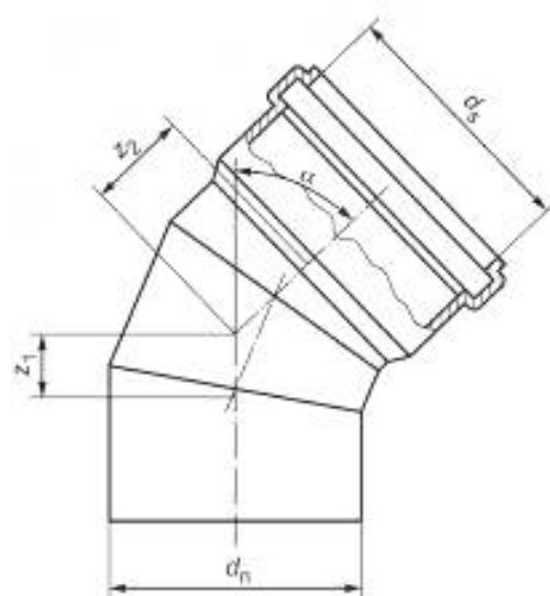
б) отвод сварной
