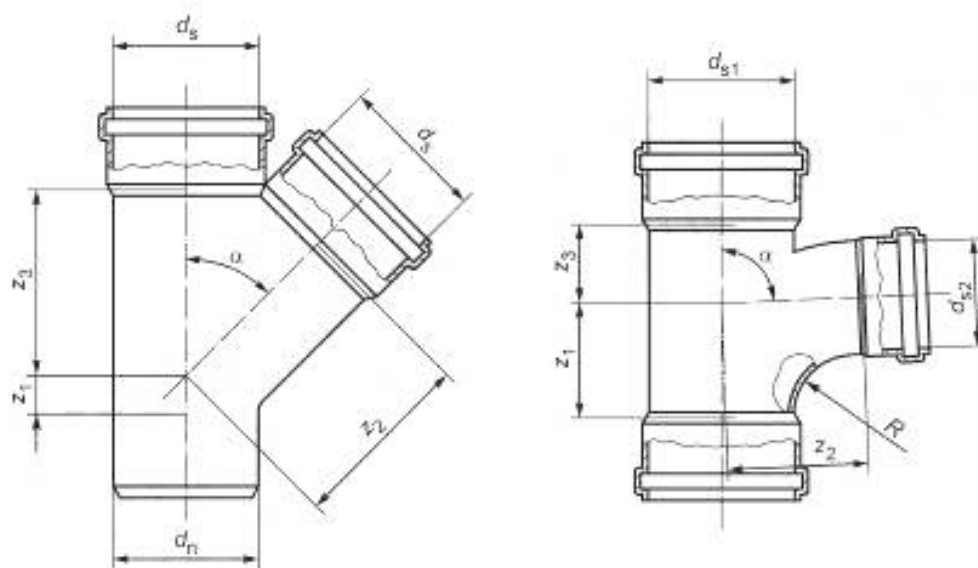
Рисунок 5 — Тройник
