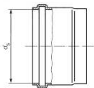
Рисунок 10 — Патрубок для стыковой сварки
