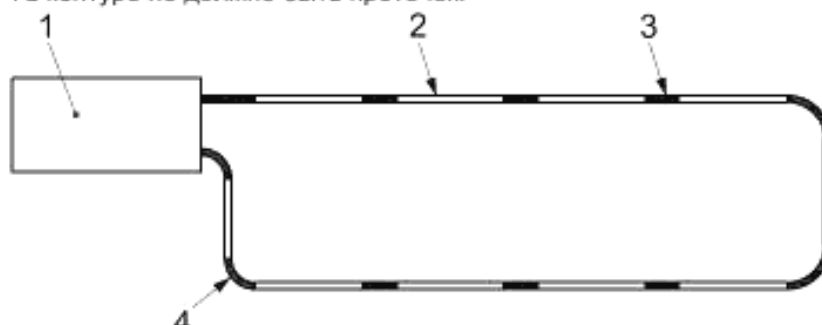
1 – ротационный насос и система нагрева; 2 – отрезки труб из PVC-C тип I длиной 300 мм; 3 – муфта PVC-C тип I; 4 – угольник PVC-C тип I
