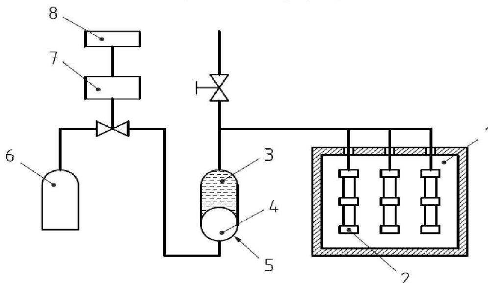
Рисунок 6 – Схема стенда для проверки стойкости соединений при переменном давлении
