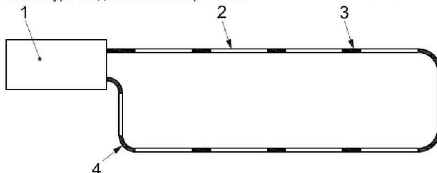
Рисунок 2 – Схема испытаний материала труб и фитингов PVC-C тип I на стойкость к аварийной температуре T_{\text{авар}}
