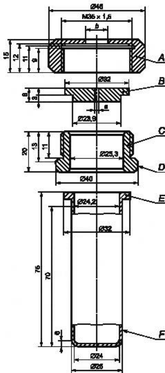
Рисунок 4 — Прибор для проведения испытания по Коенену (опытный комплект с трубкой)
