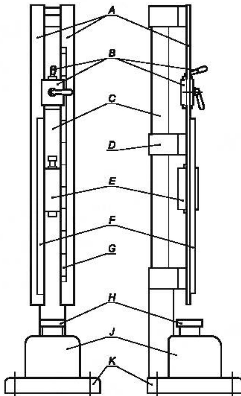
А — две направляющие рейки; В — захватно-пусковое устройство; С — стойка; D — средняя перекладина; E — падающий груз; F — зубчатая рейка; G — градуированная шкала; H — наковальня ( \varnothing 100 \times 70 мм); J — стальной блок, 230 \times 250 \times 200 мм; K — основание, 450 \times 450 \times 60 мм
