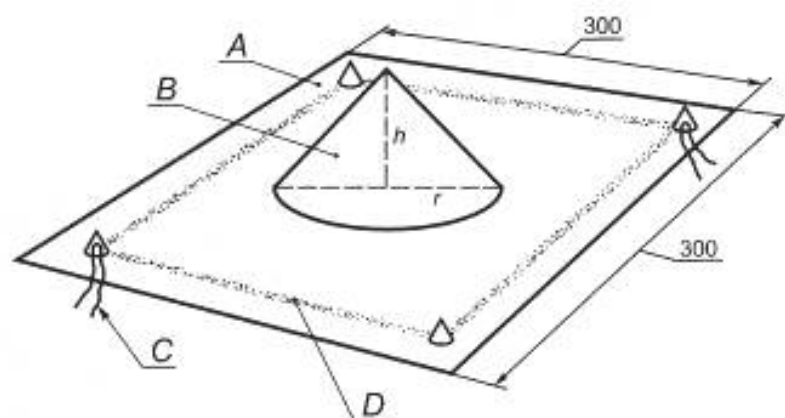
A — лист крафт-бумаги; B — испытуемая химическая продукция; C — зажигание от воспламенителя нескольких граммов мелкозернистого черного пороха (с двух противоположных углов); D — полоска мелкозернистого черного пороха
