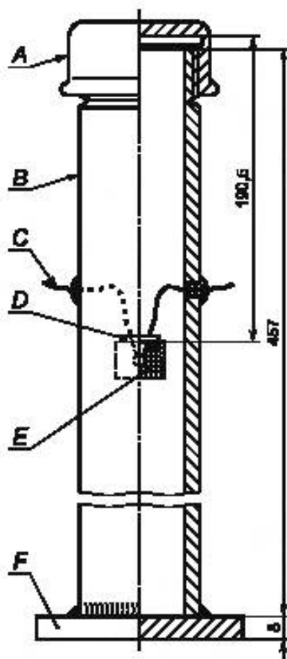
А — кованный стальной колпак; В — стальная труба; С — выводы воспламенителя; D — уплотнение; Е — комплект воспламенителя; F — контрольная плита
