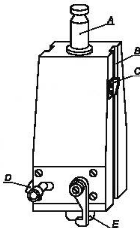
Рисунок 13 — Падающий груз
