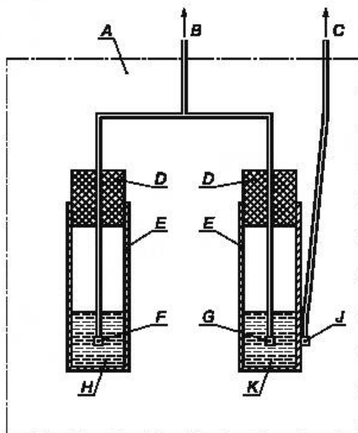
А — печь; В — к мультиметру ( T_1 - T_2 ); С — к мультиметру ( T_3 ); D — пробки; E — пробирки; F — термодар № 1 ( T_1 ); G — термодар № 2 ( T_2 ); H — 100 см 3 образца; J — термодар № 3 ( T_3 ); K — 100 см 3 эталонной химической продукции
