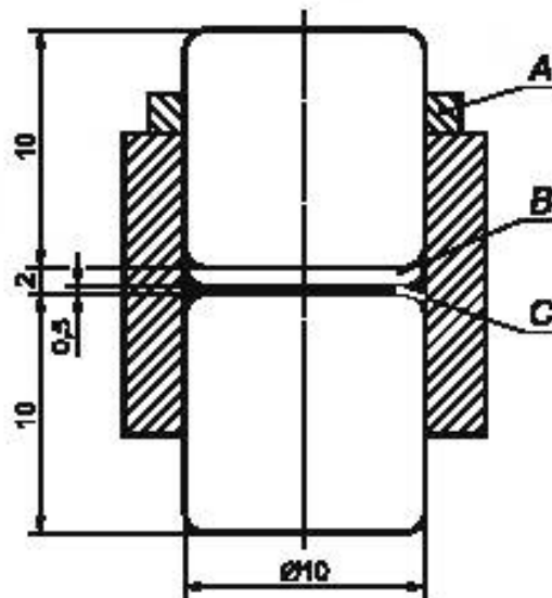
А — резиновое кольцо; В — пространство, не заполненное жидкостью; С — жидкий образец, распределенный по окружности стального цилиндра
