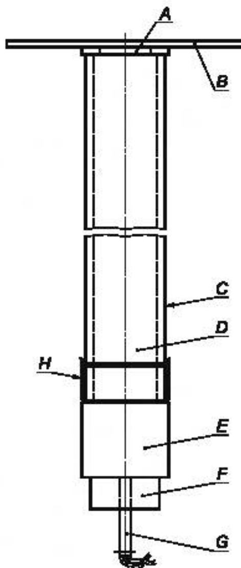
А — прокладки; В — контрольная пластина; С — стальная трубка; D — испытуемая химическая продукция; Е — бустер, состоящий из циклотриметилентринитрамина/парафина или ТЭН/тротила; F — держатель детонатора; G — детонатор; H — пластмассовая мембрана
