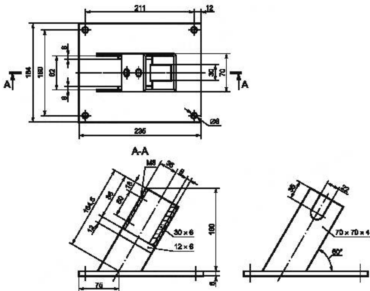
Рисунок 8 — Опорный стенд
