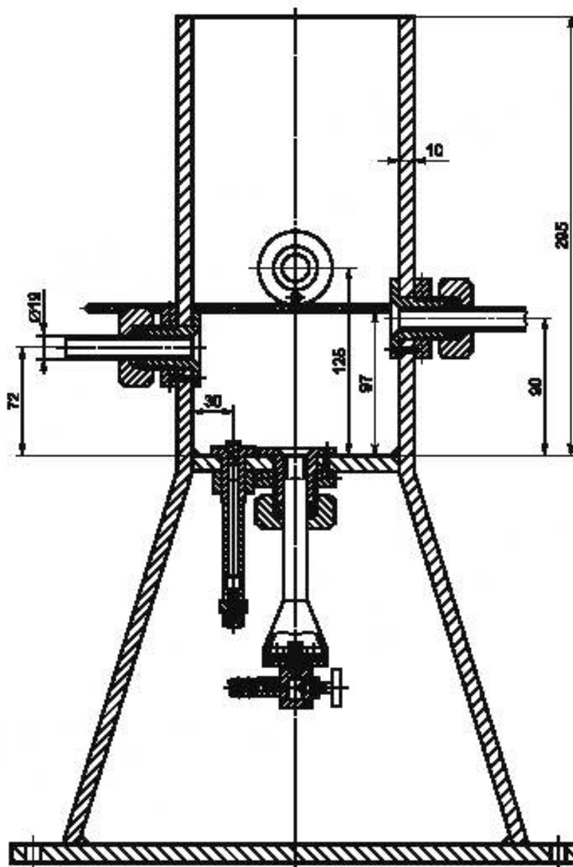
Рисунок 5 — Защитно-нагревательное устройство
