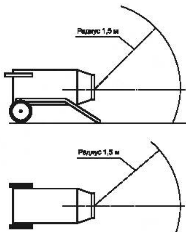
Рисунок 2 — Измерение температуры нагнетаемого воздуха
