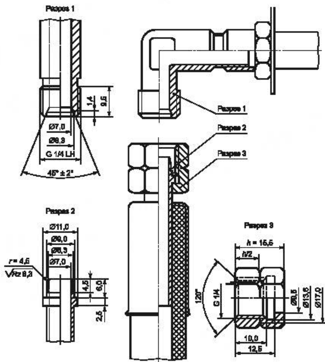
Рисунок Б.1 — Муфты для шлангов
