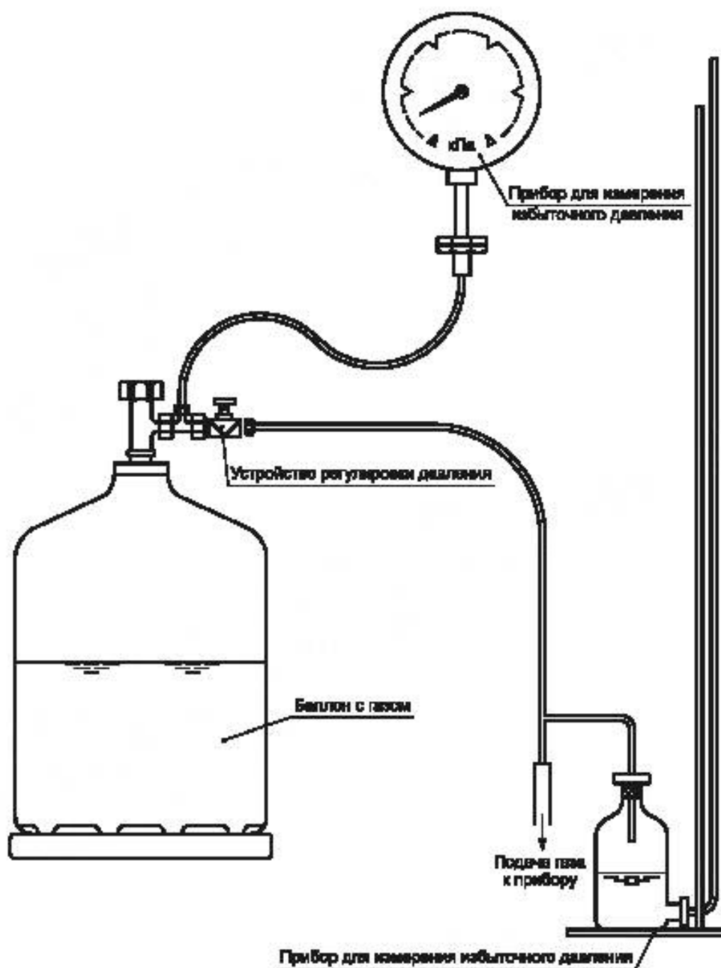
Рисунок 1 — Аппаратура для измерения повышения давления
