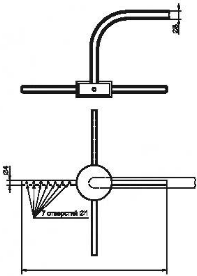
Рисунок 3 — Пробоотборник
