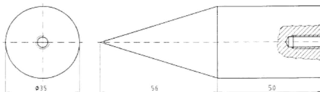
Рисунок 1 — Зонд
