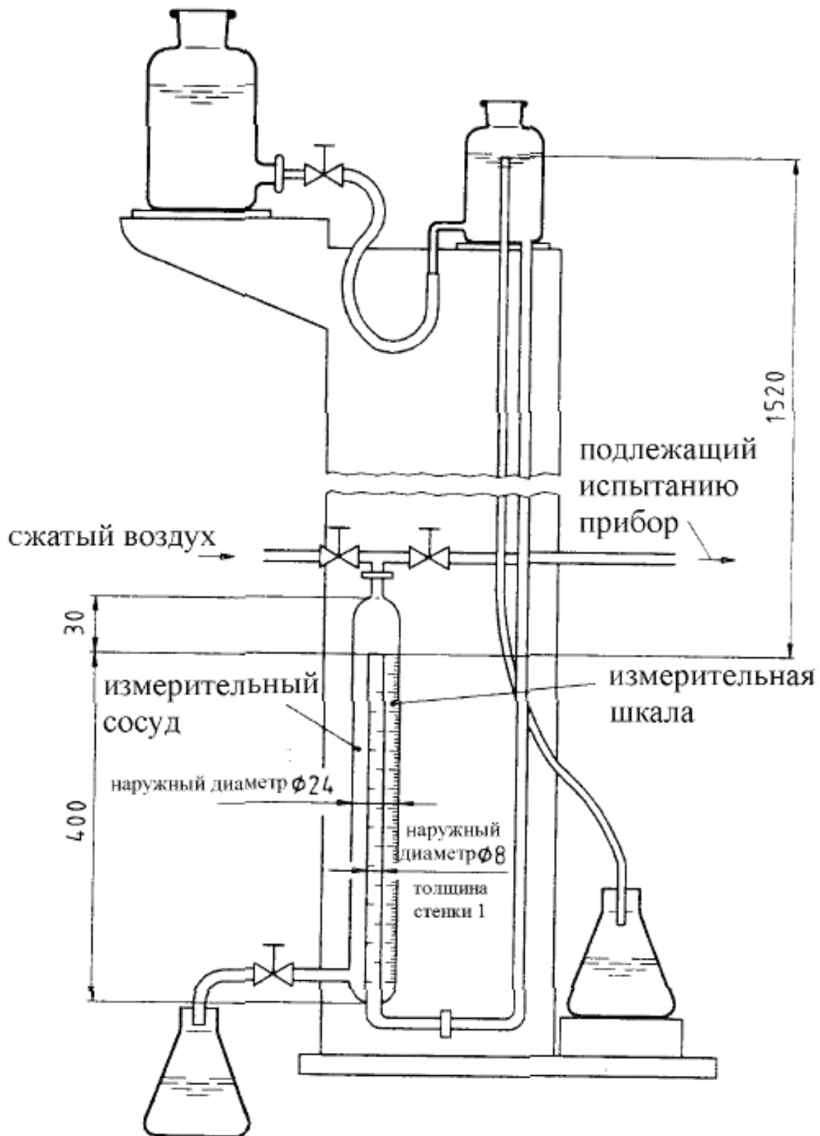
Рисунок 2 — Устройство для испытания прибора на герметичность
