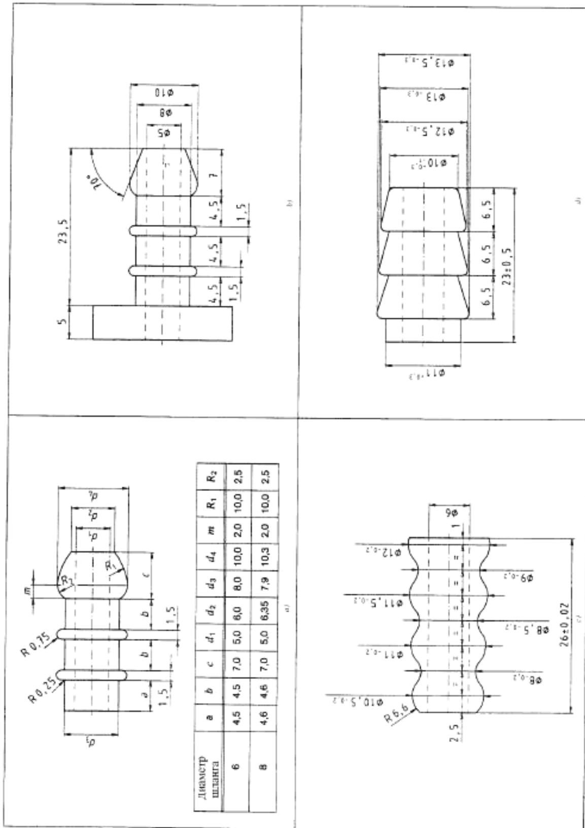
Рисунок А.1 – Присоединительные штуцеры
