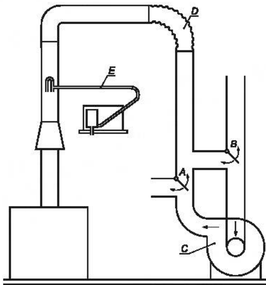
A, B — переключающие заслонки для обеспечения прямой и обратной тяги; C — вентилятор; D — гибкий патрубок; E — измерение скорости потока при помощи трубки Пито
