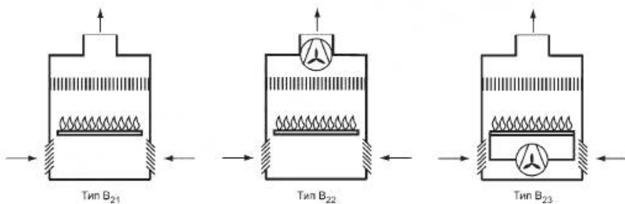
Рисунок В.2 — Схемы приборов типа В 2
