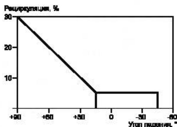
Рисунок С.1 — Максимальная допустимая рециркуляция продуктов сгорания
