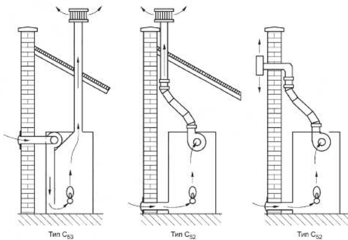
Рисунок В.5 — Схемы приборов типа C 5
