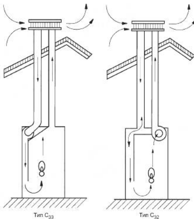
Рисунок В.4 — Схемы приборов типа C 3
