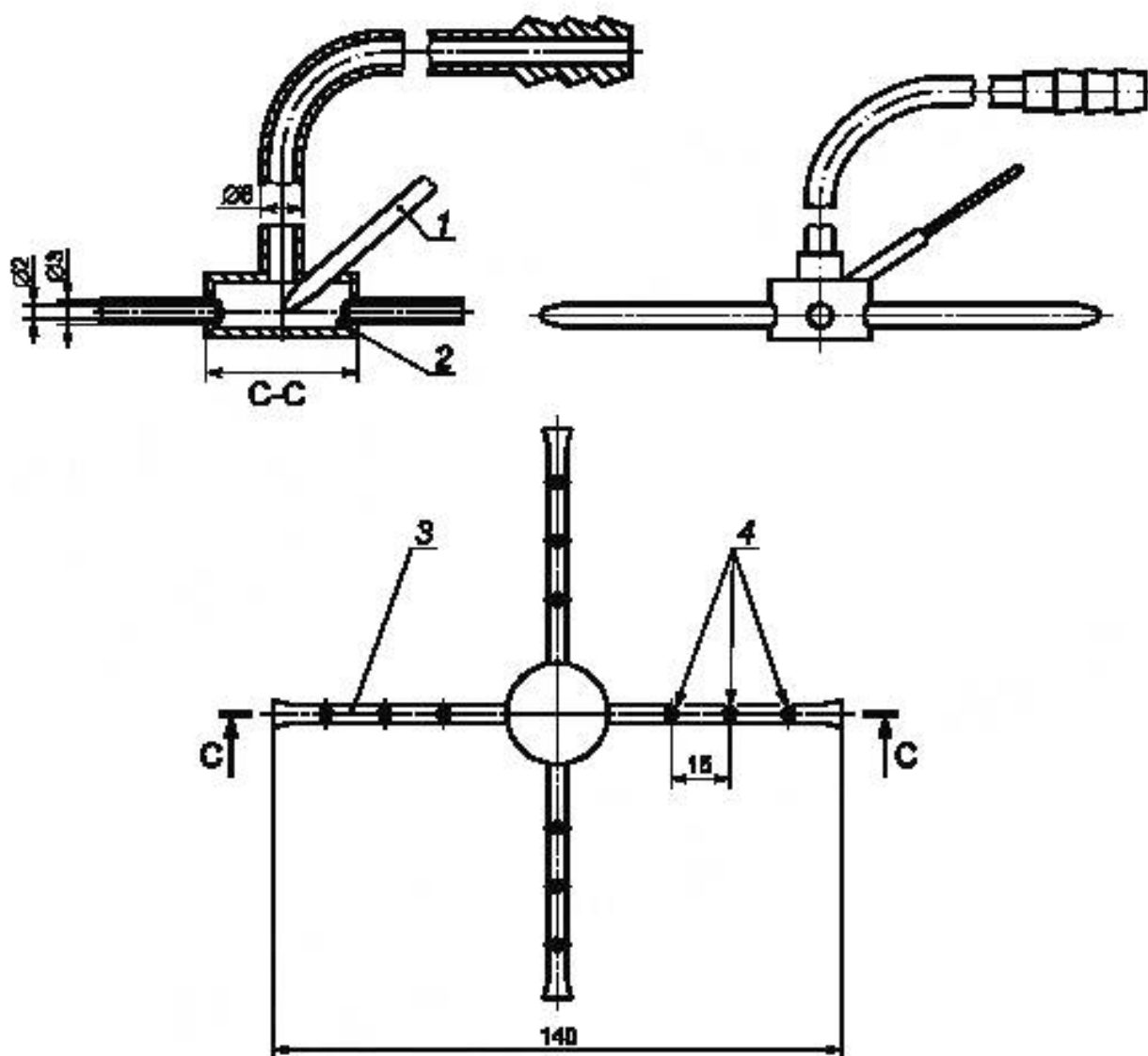
1 — трубка с двумя каналами, в которых расположены провода термодпары; 2 — точка измерения температуры; 3 — трубка с глухим концом; 4 — отверстия
