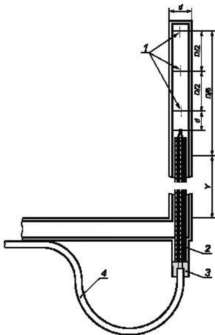
1 — точки отбора проб; 2 — керамическая трубка с двумя каналами; 3 — изолирующий цемент; 4 — провода термопары (хромель — алюмель)
