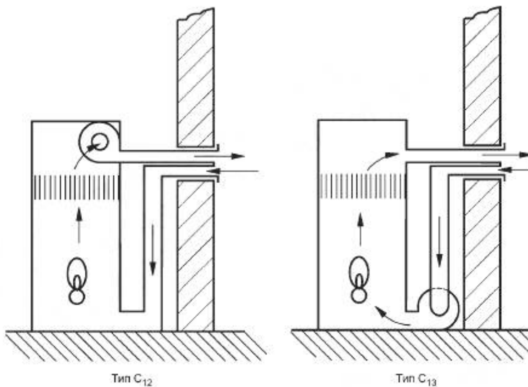
Рисунок В.3 — Схемы приборов типа C 1
