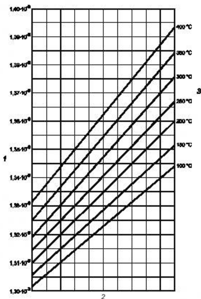
Рисунок 12 — Средняя удельная теплоемкость продуктов сгорания
