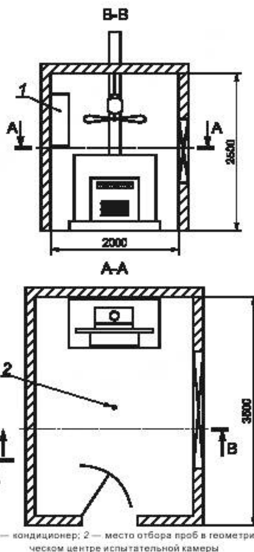
Рисунок 6 — Камера для испытания устройства контроля воздуха в помещении
