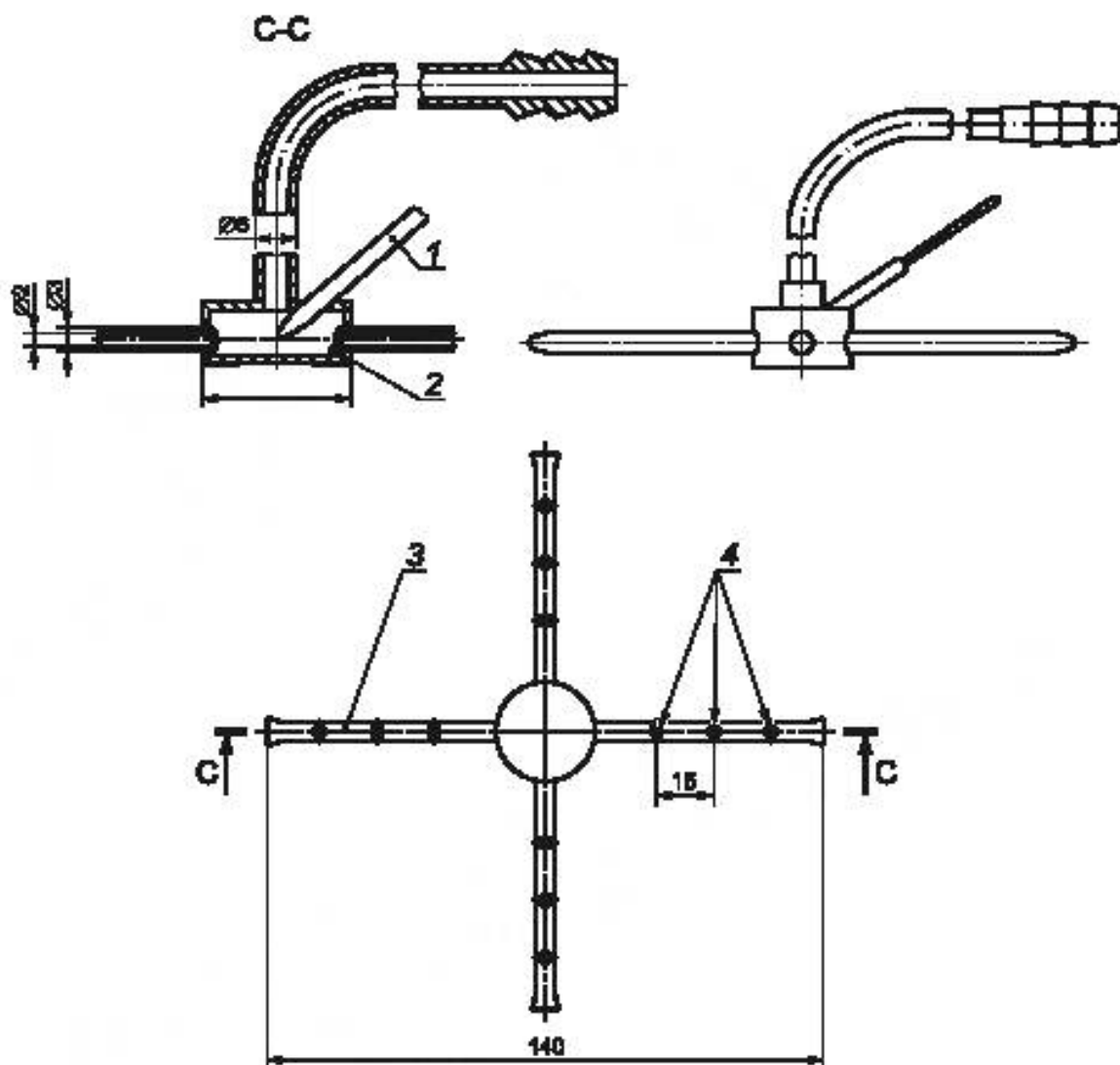
1 — трубка с двумя каналами, в которых расположены провода термпары; 2 — точка измерения температуры; 3 — трубка с глухим концом; 4 — отверстия
