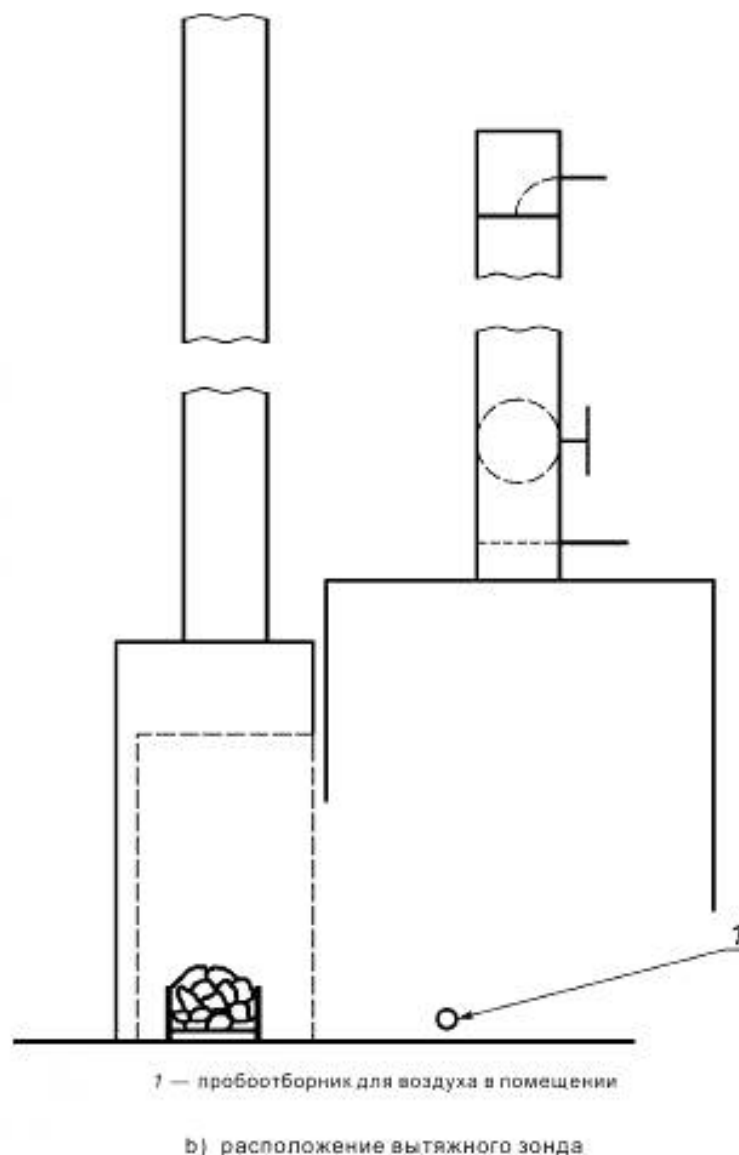
Рисунок 2 — Вытяжной зонд
