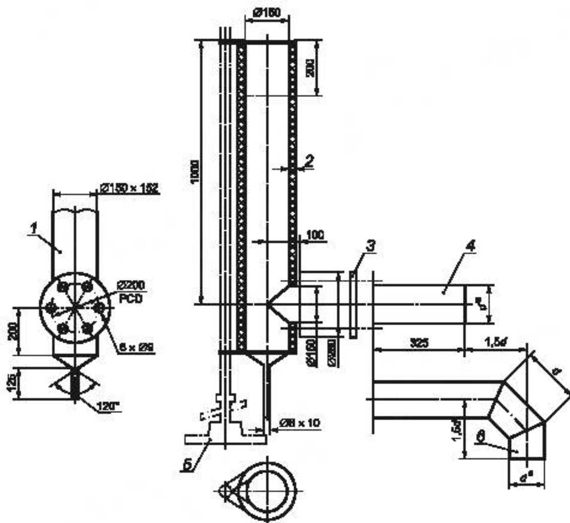
1 — труба дымохода из нержавеющей стали; 2 — теплоизоляция (стекловолно плотностью 84 \text{ кг/м}^3 ); 3 — прокладка; 4 — соединительная труба из нержавеющей стали; 5 — опорная стойка; 6 — соединительная труба из нержавеющей стали
