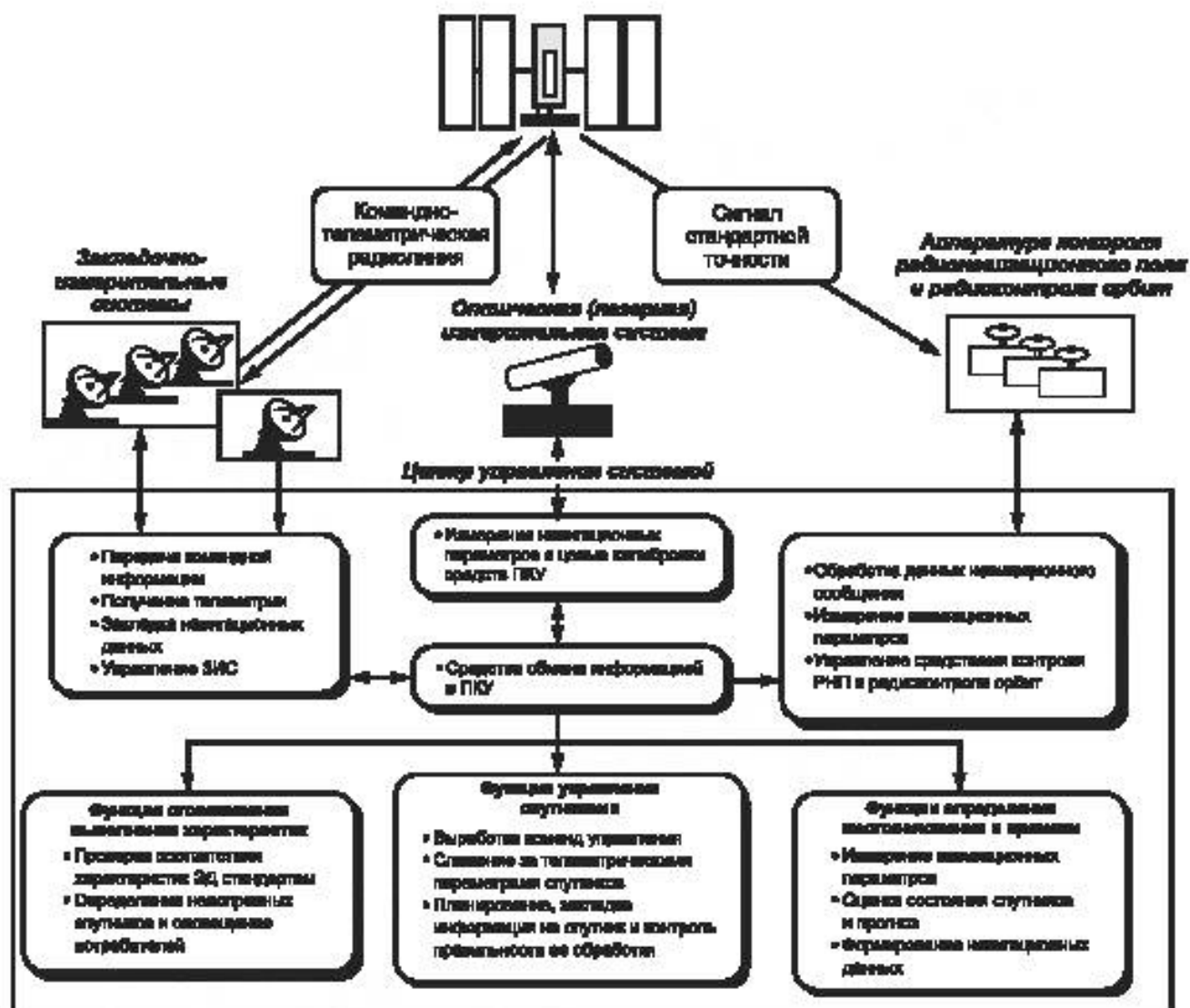
Рисунок А.2 — Процесс управления системой спутников
