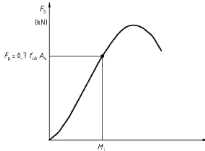
Рисунок 3 — Диаграмма «крутящий момент — усилие натяжения»
