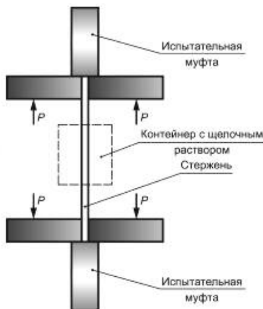
Рисунок 6.1 — Схема испытания образцов на длительную прочность
